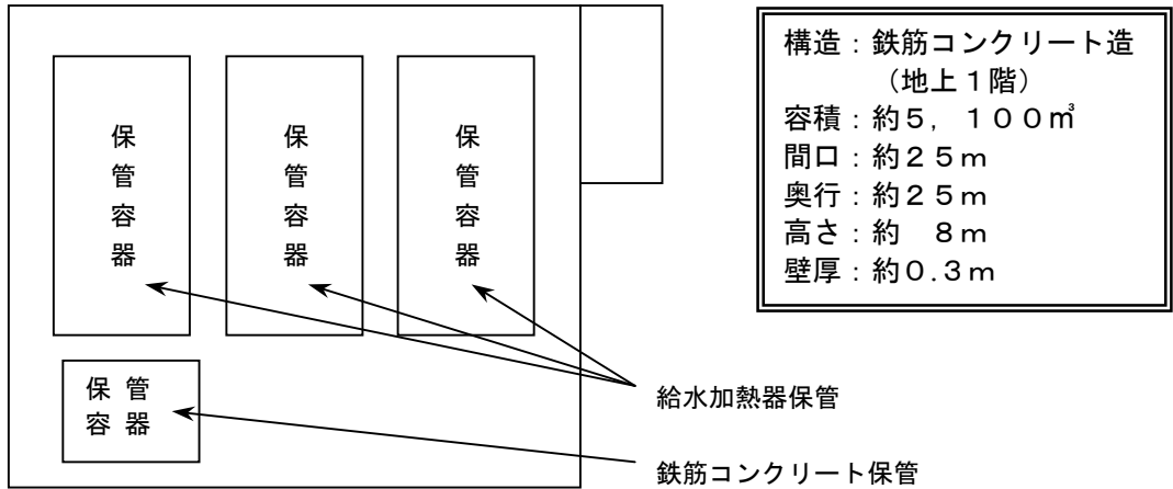
建屋平面図
