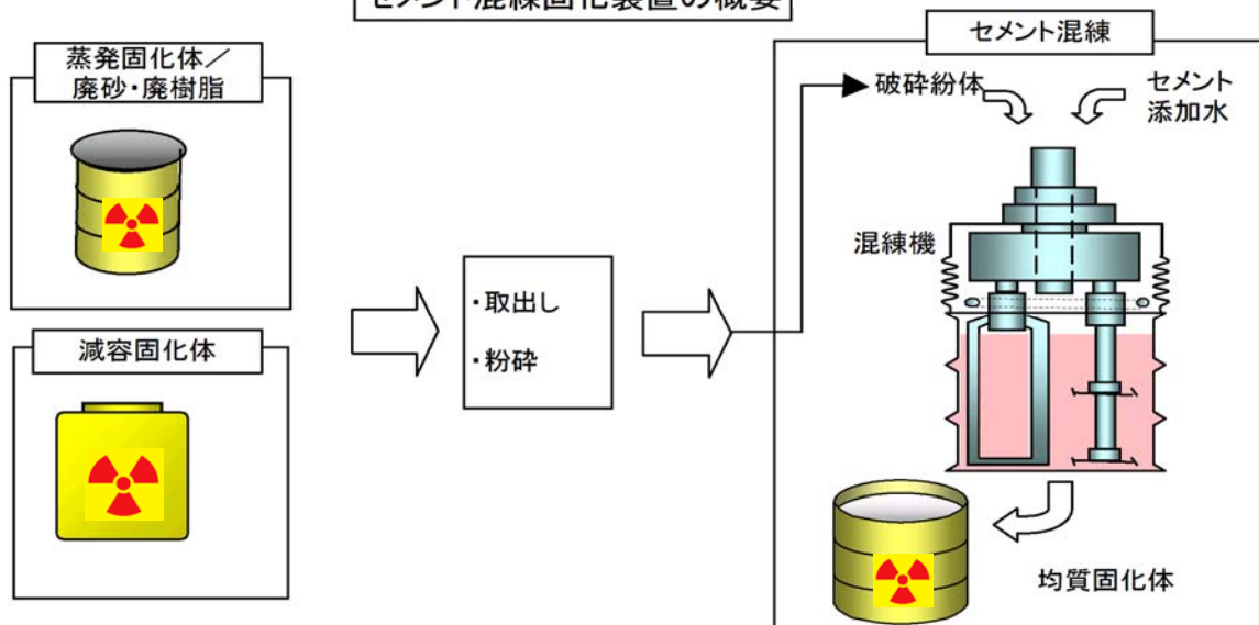
セメント混練固化装置の概要
