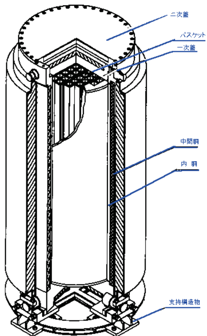
第3図 使用済燃料乾式貯蔵容器及び支持構造物の概要図
