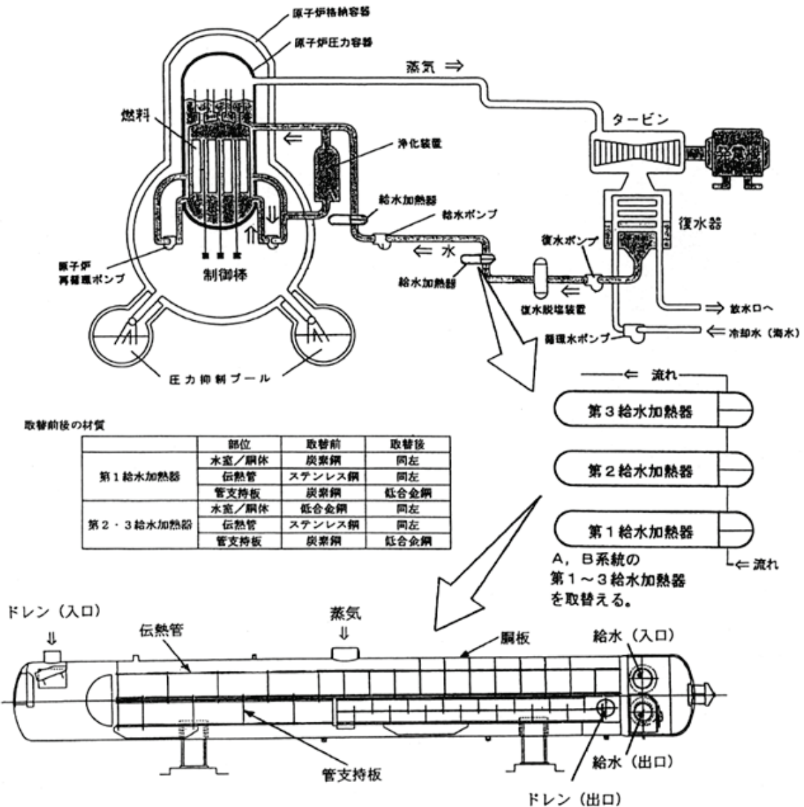
給水加熱器仕様
