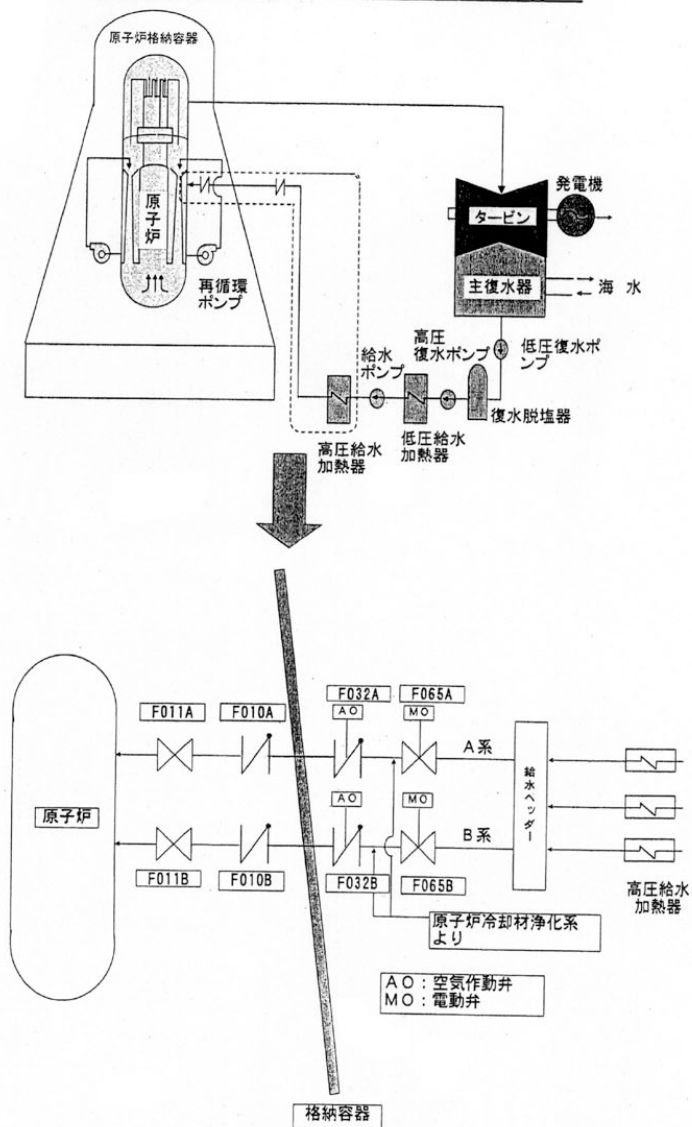
原子炉給水系統概略図
