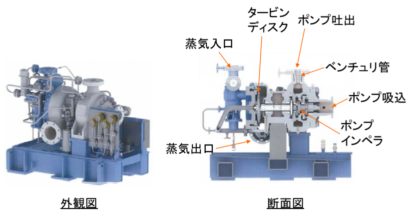
図－ 9 高圧代替注水ポンプ構造概要
