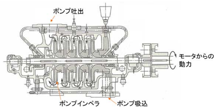
図－ 7 多段ポンプ構造図例
