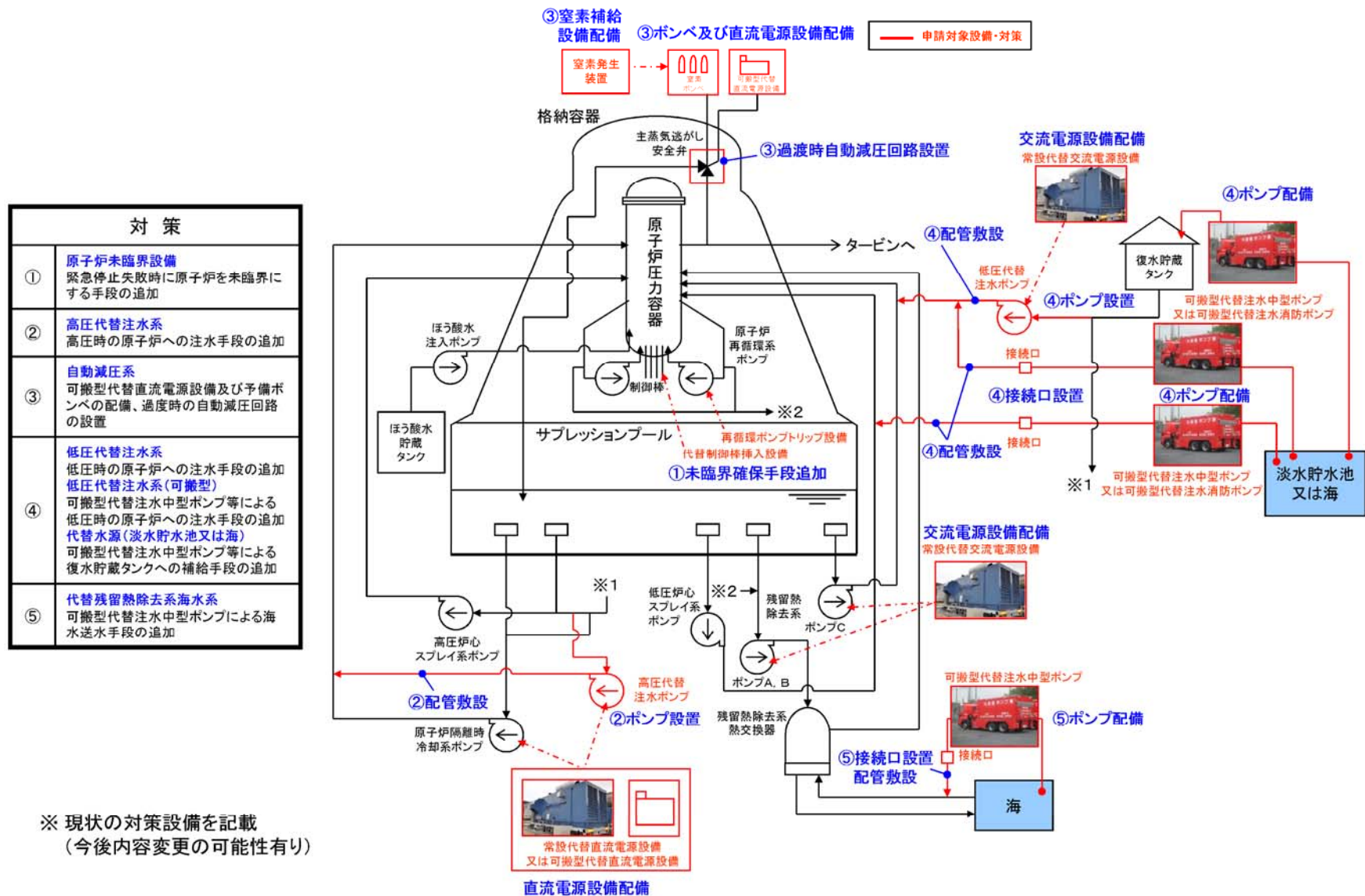
図－3 炉心損傷防止対策全体概要
