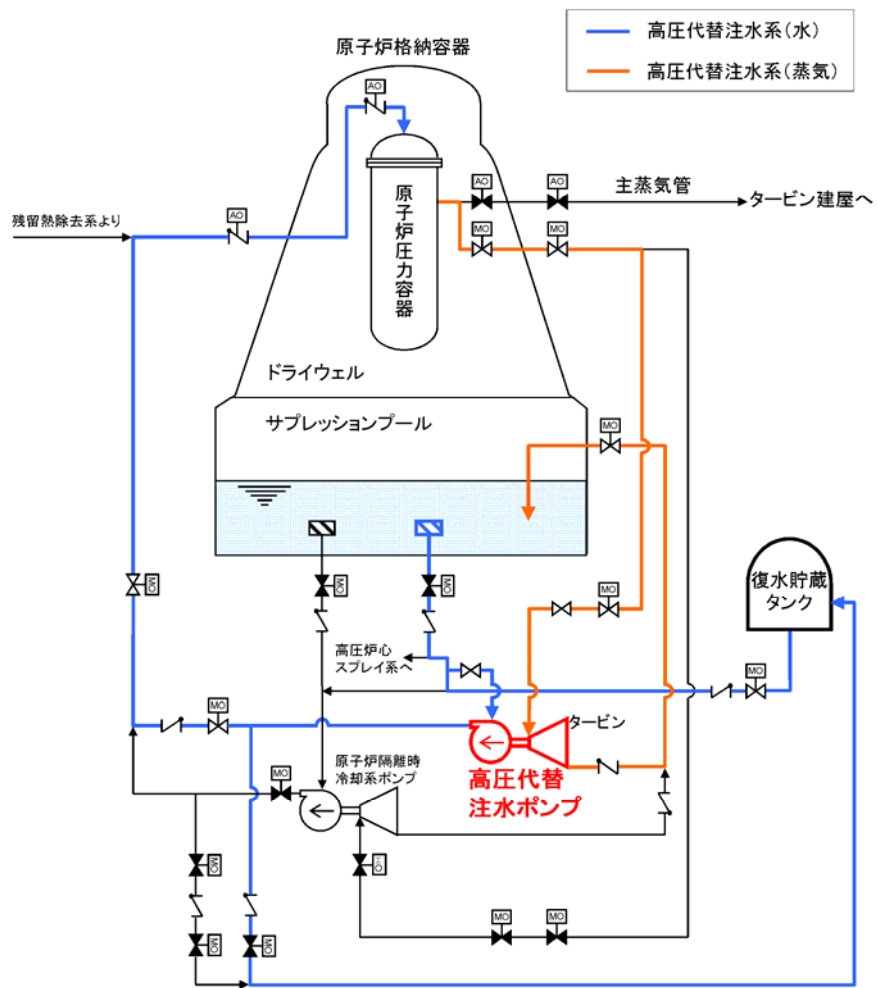
図－ 8 高圧代替注水系概要
