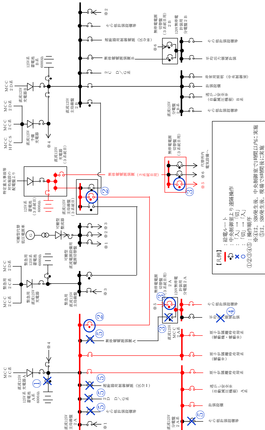
第 57-4-2 図 所内常設直流電源設備（3 系統目）から給電される系統（A 系統給電の場合）
