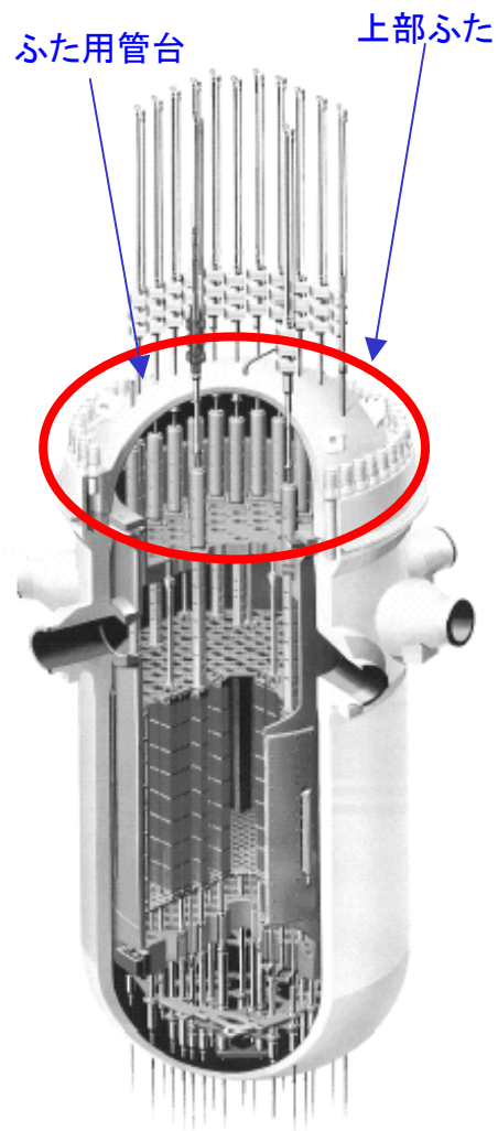
原子炉容器概要図
