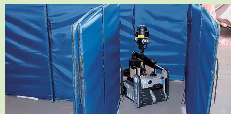
カメラを搭載した支援ロボットで現場の情報を収集する訓練(発電所建屋内の狭い空間を模擬)
