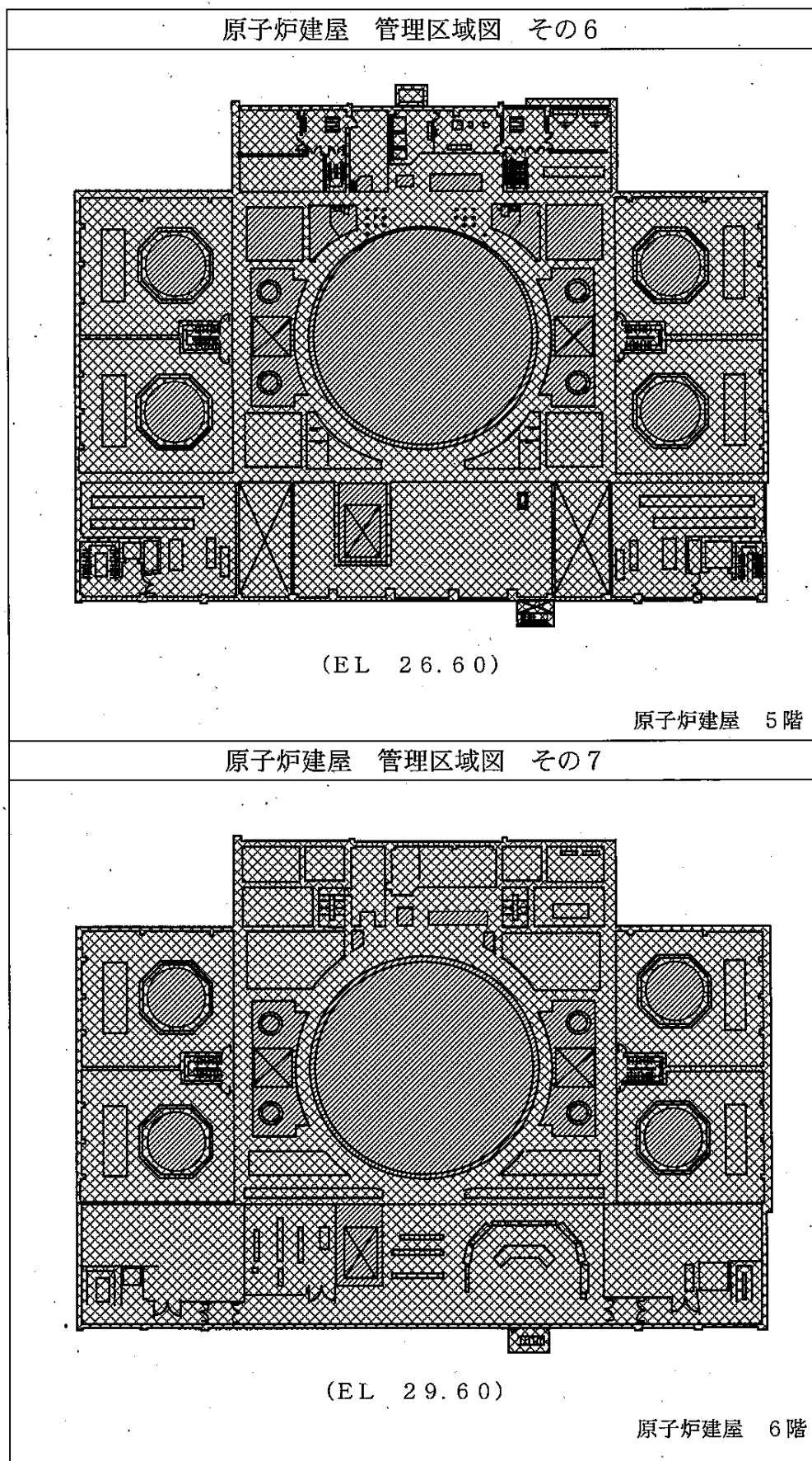
図3-1-1 廃止措置対象施設の管理区域図（廃止措置計画認可申請時点）（4/17）
