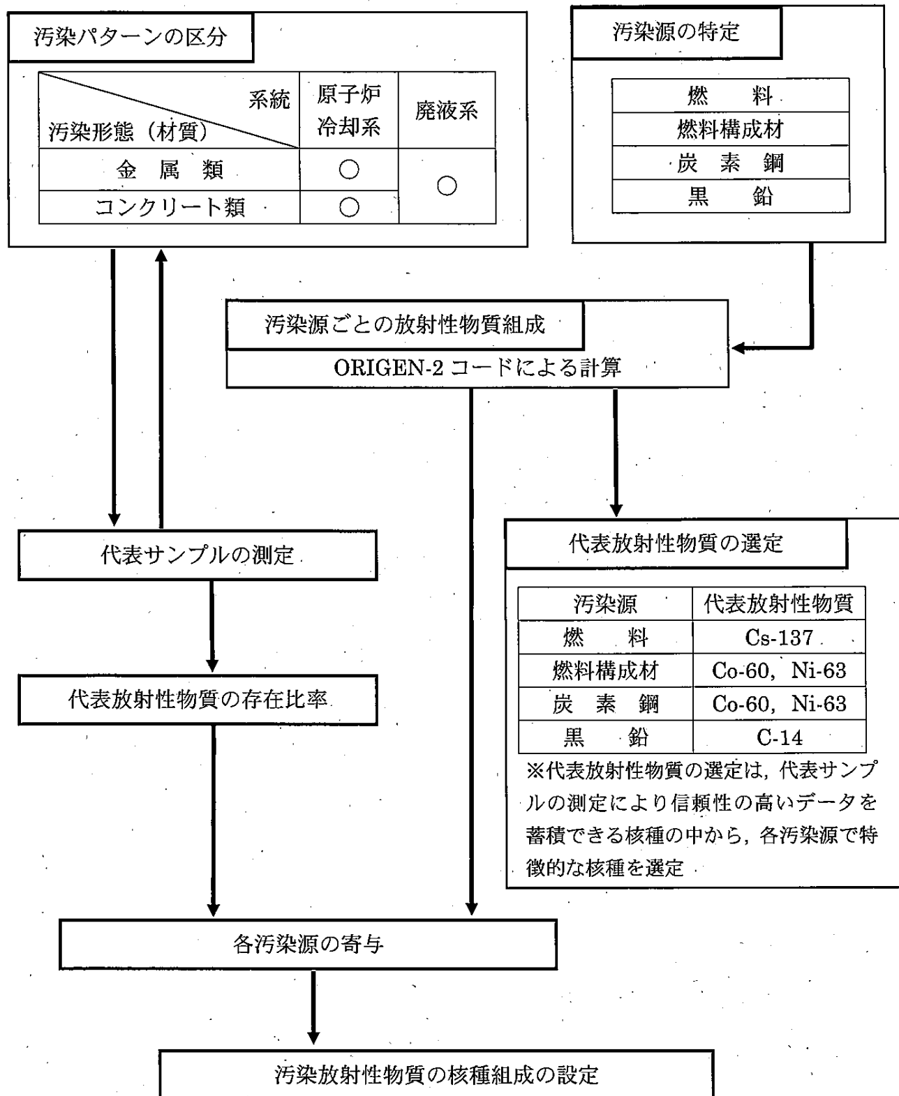
図5-3-3 放射性核種組成の設定手順
