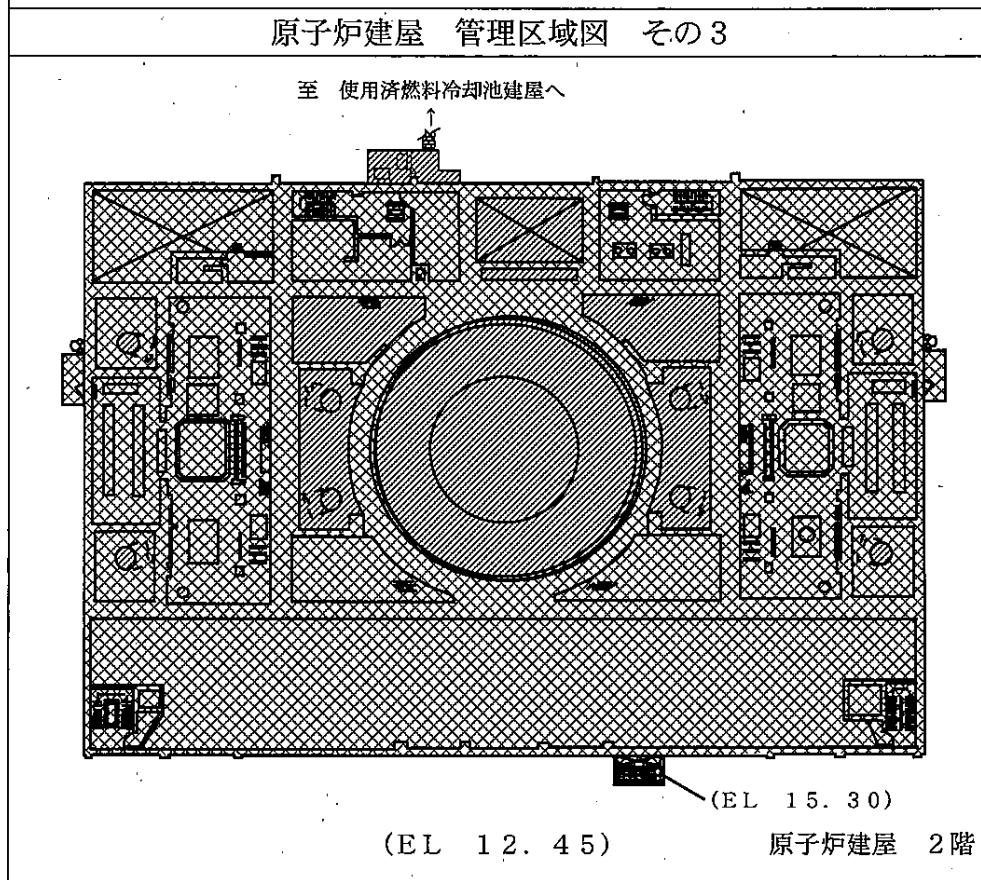
図3-1-1 廃止措置対象施設の管理区域図（廃止措置計画認可申請時点）（2/17）
