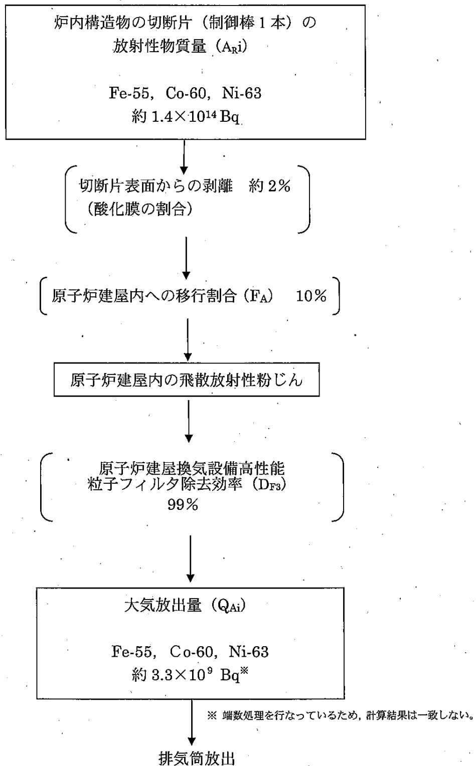
図 4 - 1 - 1 炉内構造物切断片の破損時における放射性物質の大気放出過程
