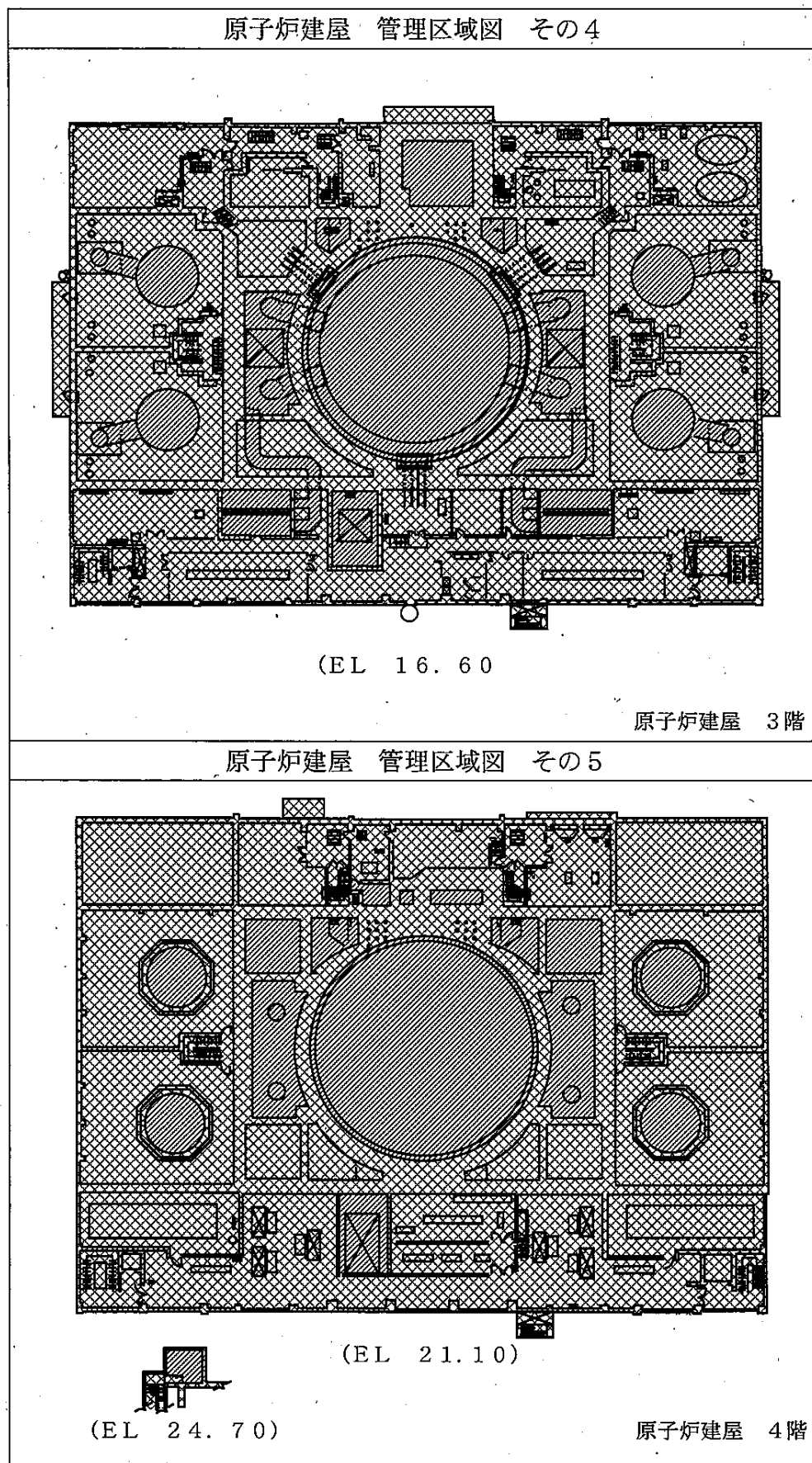
図3-1-1 廃止措置対象施設の管理区域図（廃止措置計画認可申請時点）（3/17）
