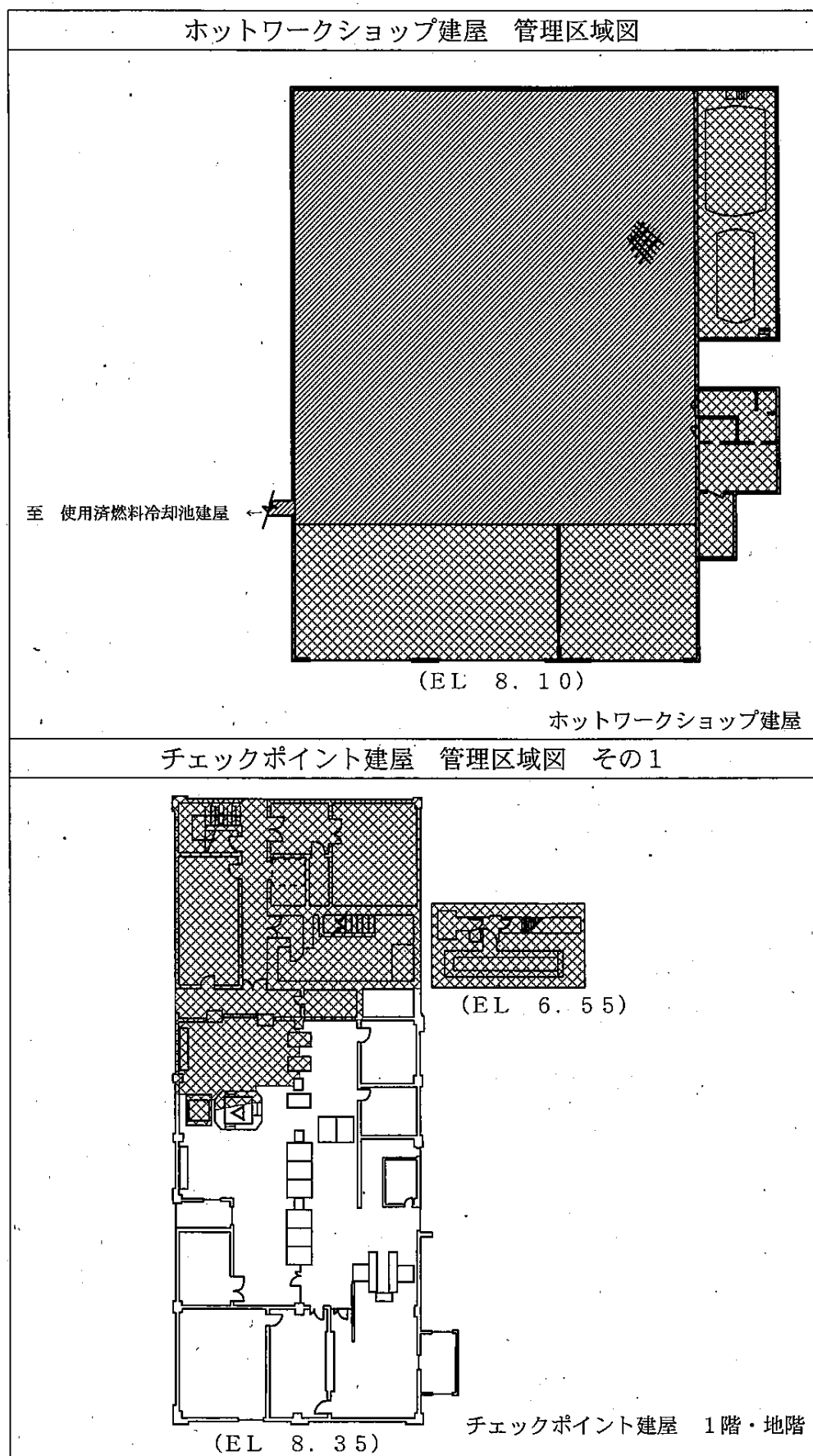
図3-1-1 廃止措置対象施設の管理区域図（廃止措置計画認可申請時点）（13/17）
