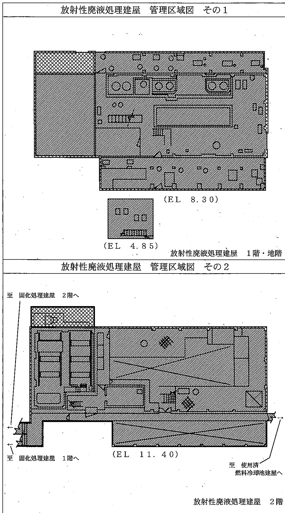
図3-1-1 廃止措置対象施設の管理区域図（廃止措置計画認可申請時点）（10/17）
