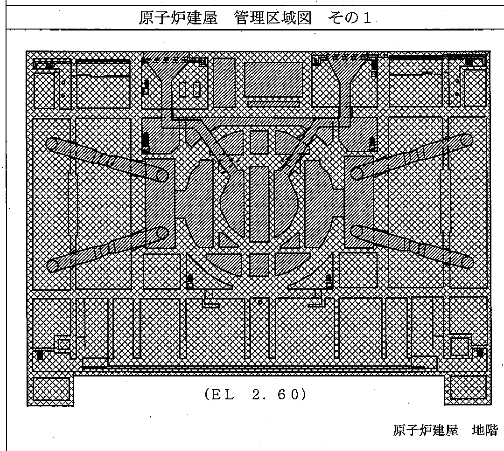
図3-1-1 廃止措置対象施設の管理区域図（廃止措置計画認可申請時点）（1／17）
