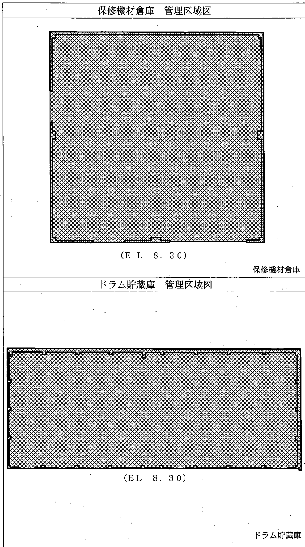
図3-1-1 廃止措置対象施設の管理区域図（廃止措置計画認可申請時点）（15／17）
