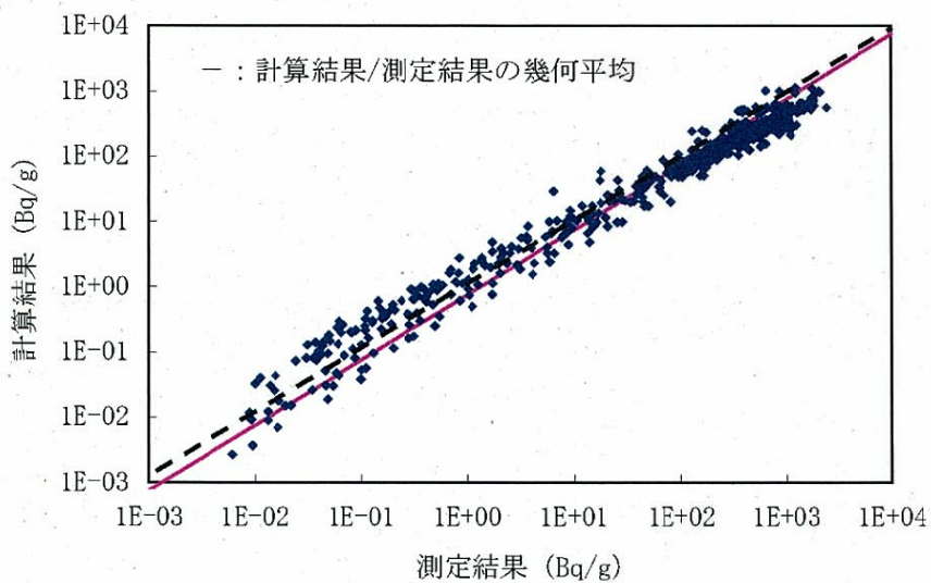
図5-2-4 放射化計算結果と測定結果の比較
