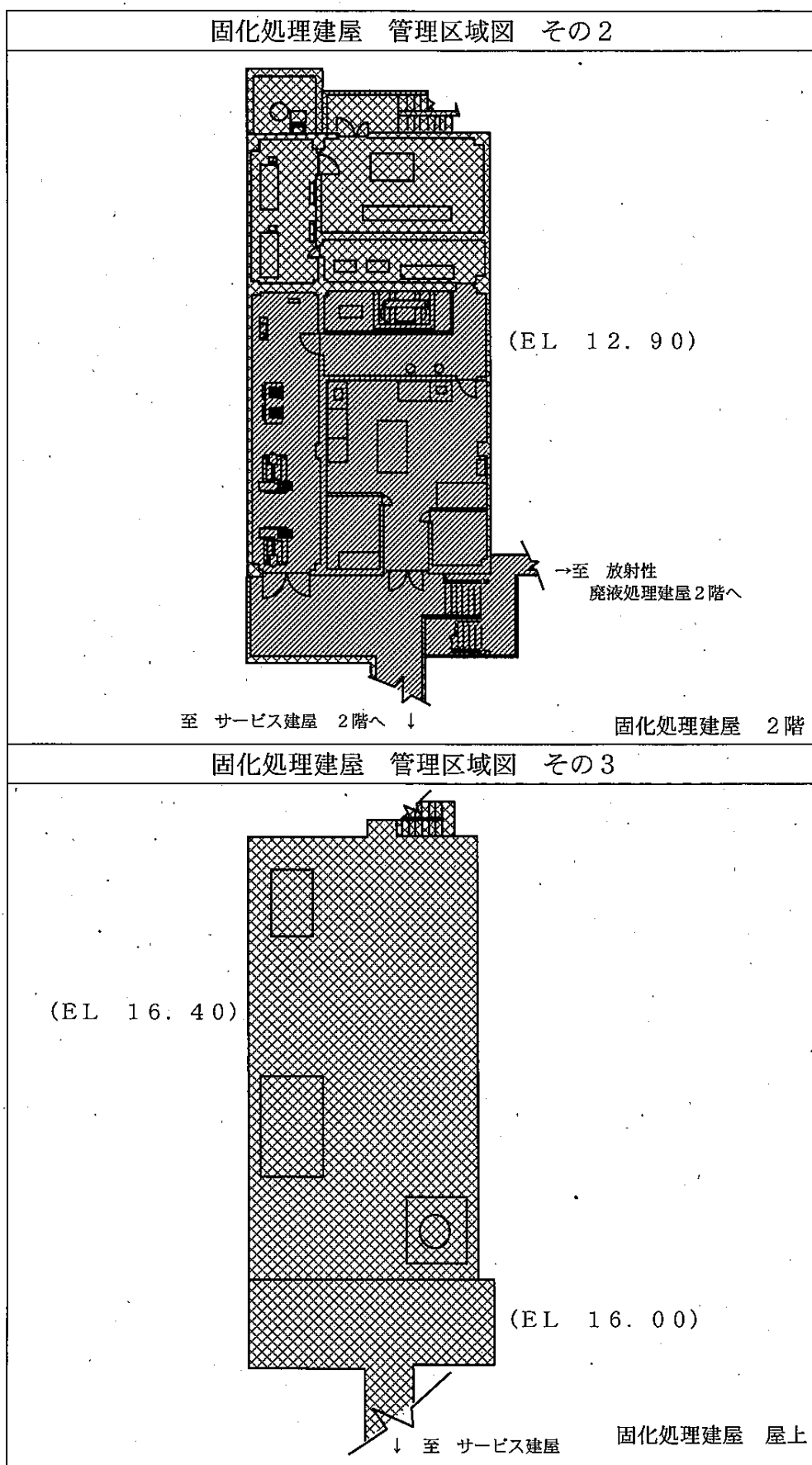
図3-1-1 廃止措置対象施設の管理区域図（廃止措置計画認可申請時点）（12/17）
