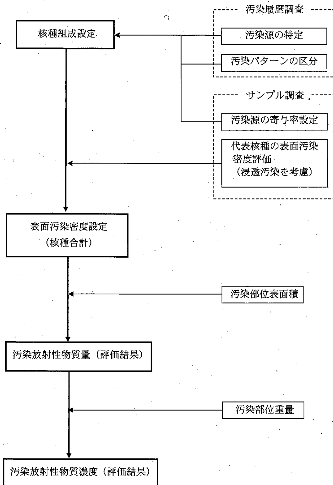
図 5 - 3 - 1 汚染放射性物質の評価手順
