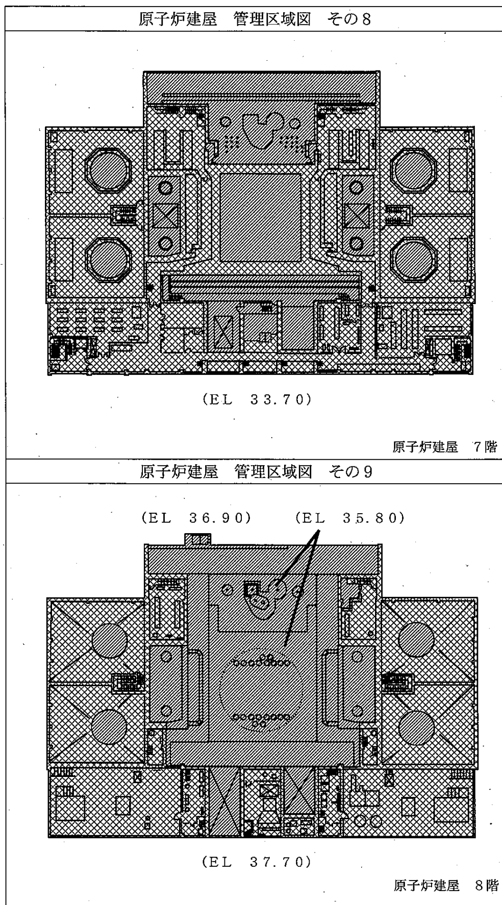
図3-1-1 廃止措置対象施設の管理区域図（廃止措置計画認可申請時点）（5/17）
