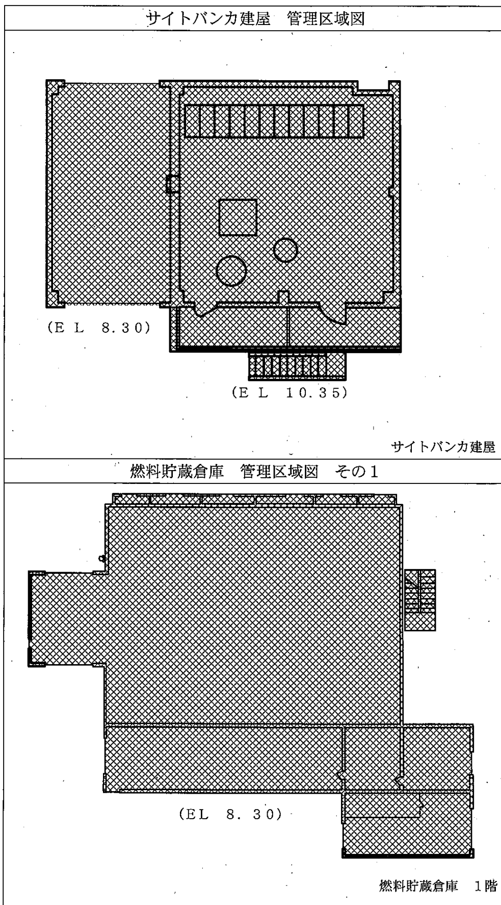
図3-1-1 廃止措置対象施設の管理区域図（廃止措置計画認可申請時点）（16／17）
