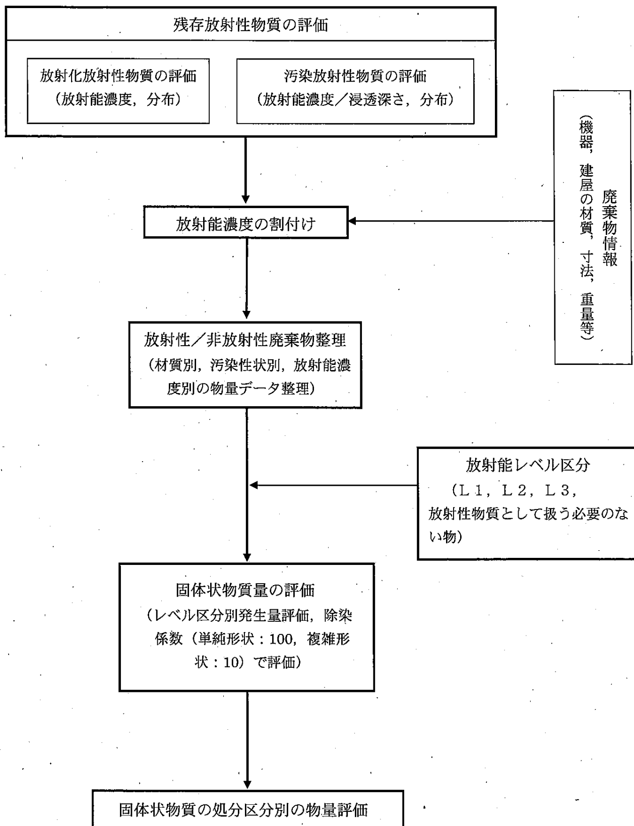
図5-5-1 核燃料物質によって汚染された固体状物質量の評価手順
