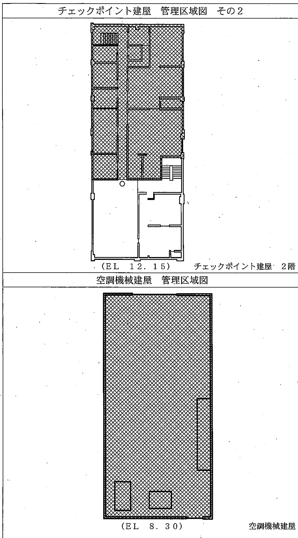
図3-1-1 廃止措置対象施設の管理区域図（廃止措置計画認可申請時点）（14/17）
