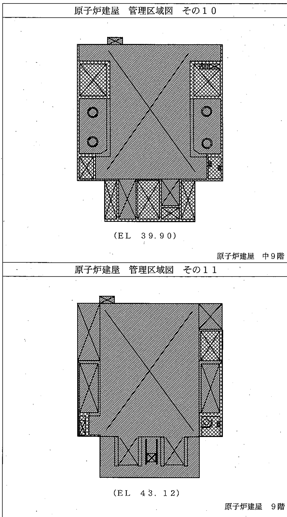
図 3 - 1 - 1 廃止措置対象施設の管理区域図（廃止措置計画認可申請時点）（6 / 17）
