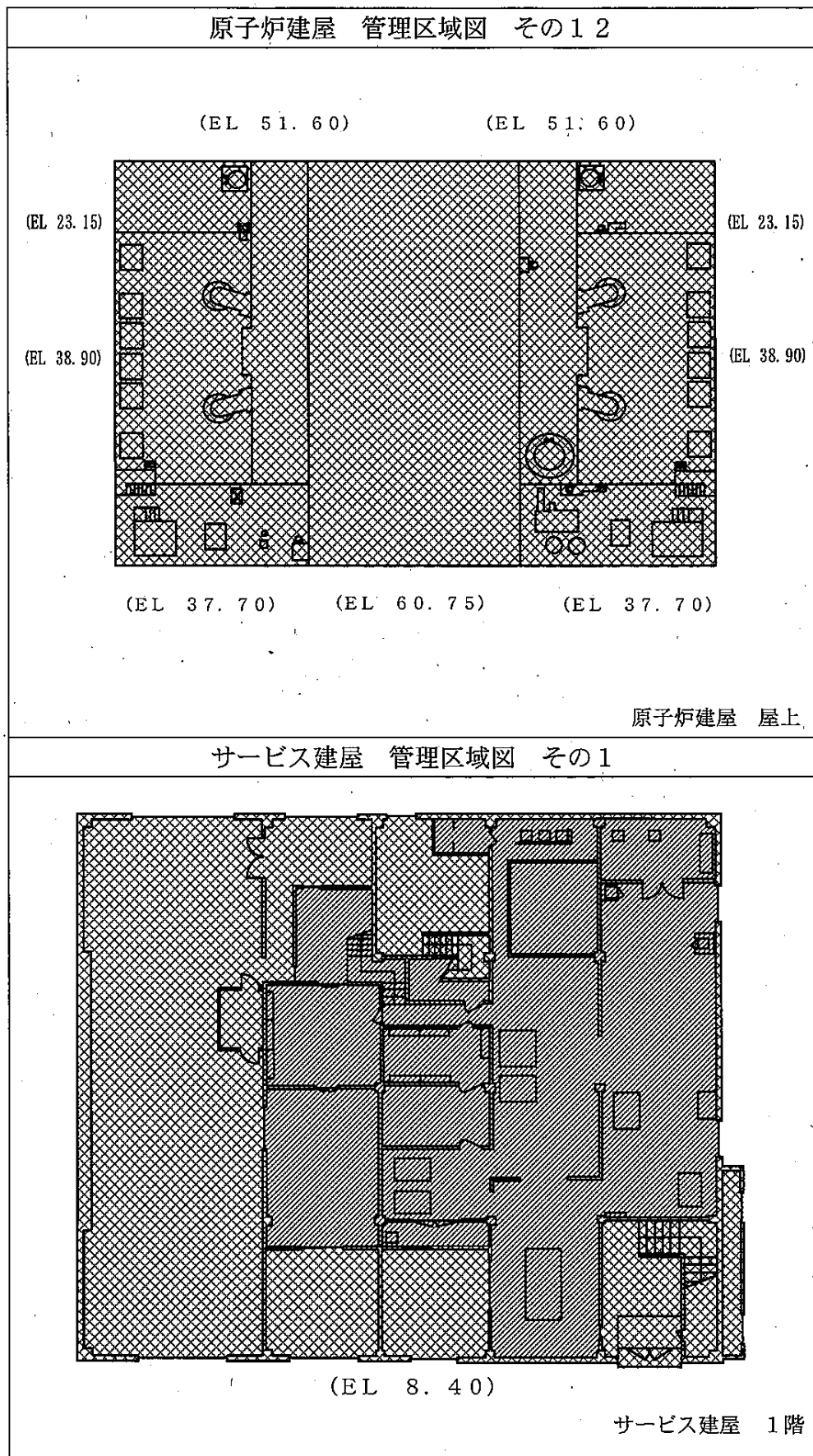
図3-1-1 廃止措置対象施設の管理区域図（廃止措置計画認可申請時点）（7/17）
