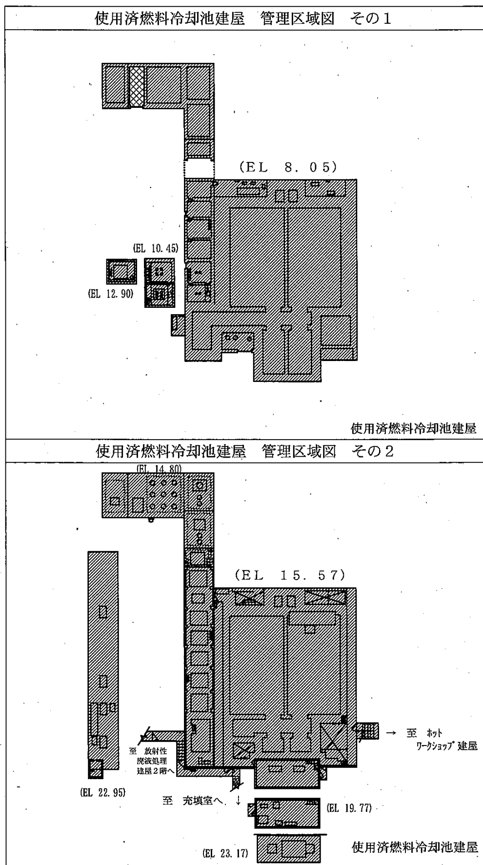
図3-1-1 廃止措置対象施設の管理区域図（廃止措置計画認可申請時点）（9/17）
