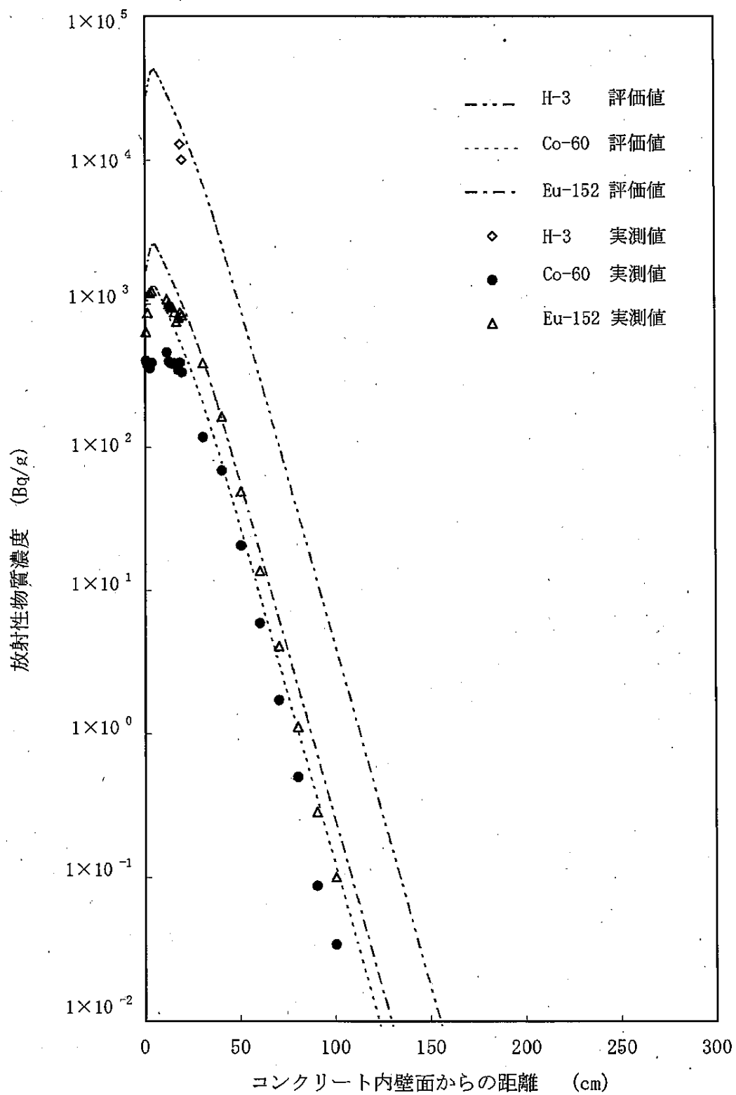
図5-2-5 生体遮へい体コンクリート壁中の放射性物質の濃度分布
