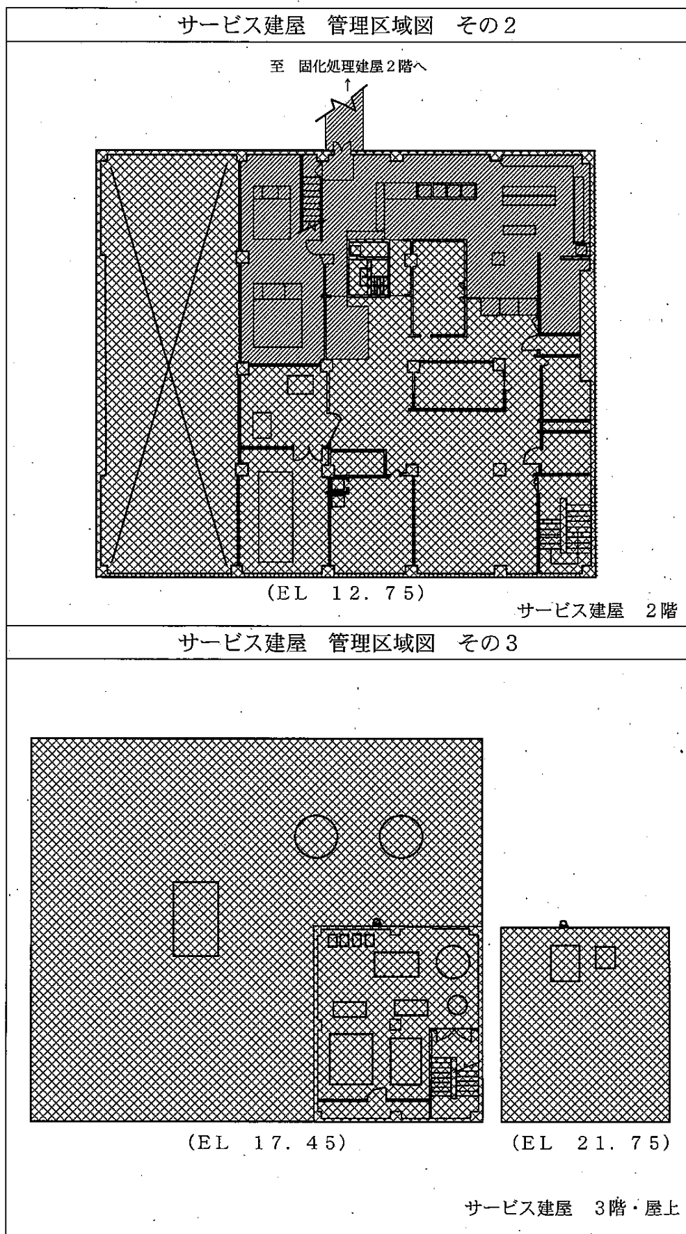
図3-1-1 廃止措置対象施設の管理区域図（廃止措置計画認可申請時点）（8/17）
