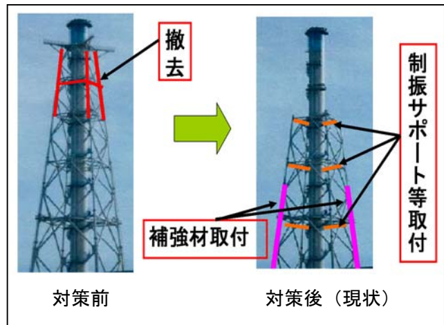
主排気筒補強工事の概要
