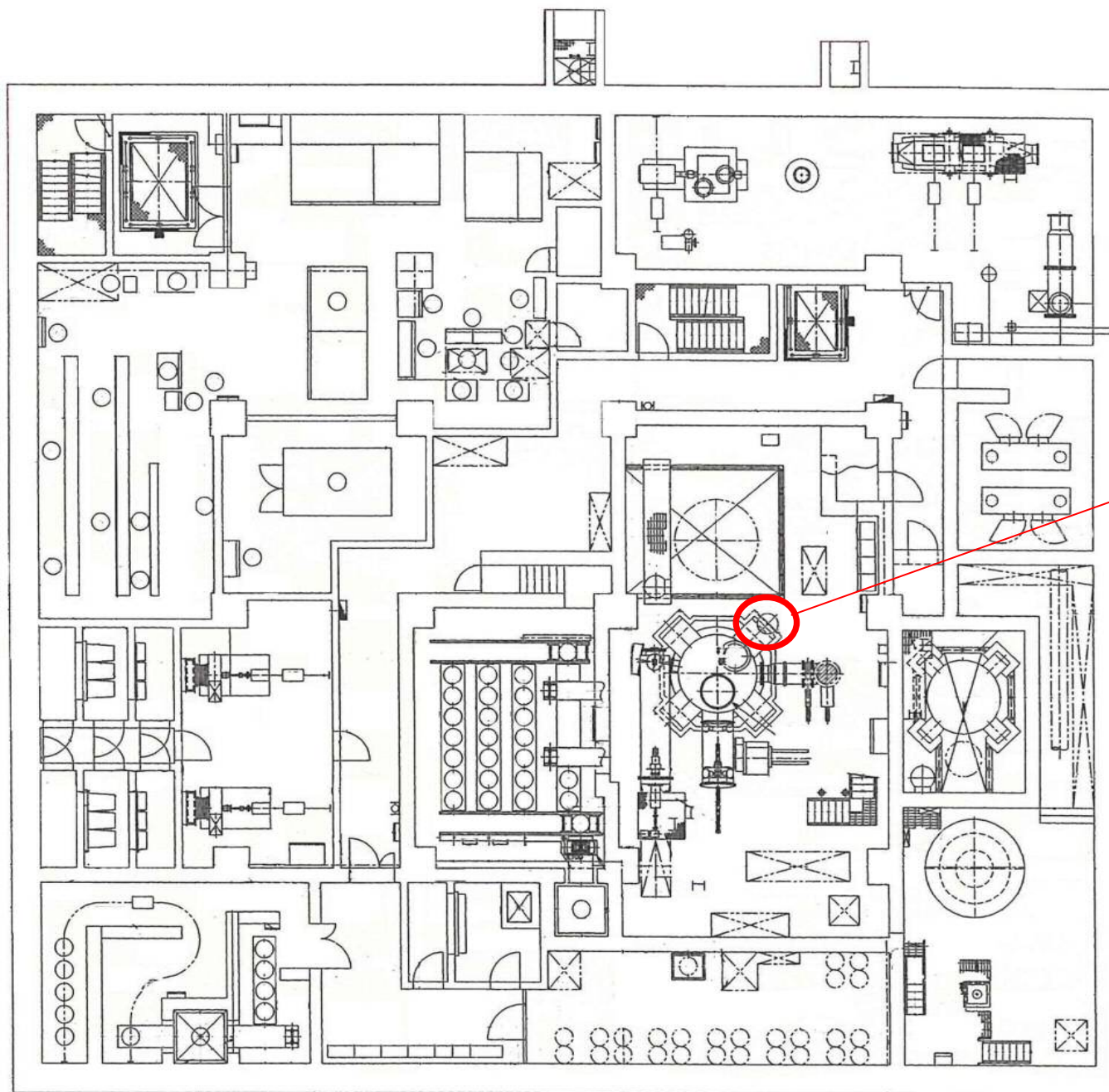
雑固体減容処理設備建屋 地下1階
