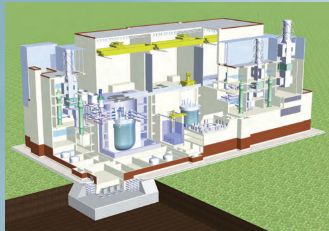
実用化段階の高速炉プラントのイメージ図 (9電力会社、電源開発(株)および当社が実施したFBR電力共通研究より)
