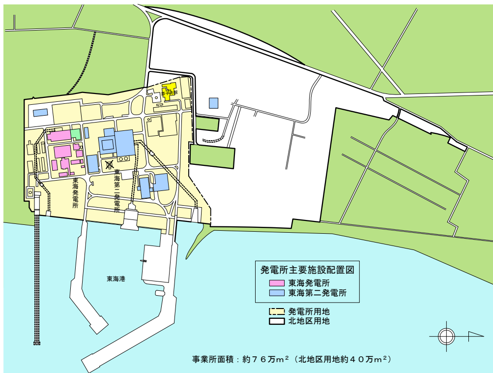
東海発電所・東海第二発電所 一般配置図
