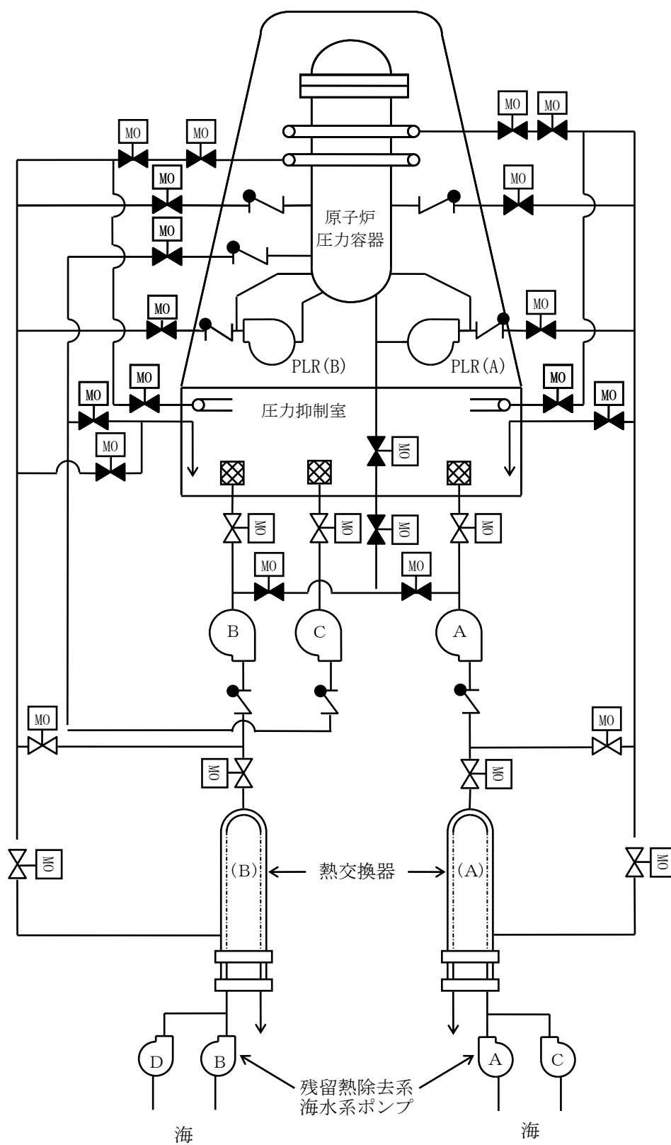
東海第二発電所 残留熱除去系 系統構成図
