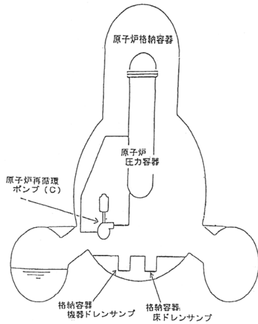
系 統 概 略 図
