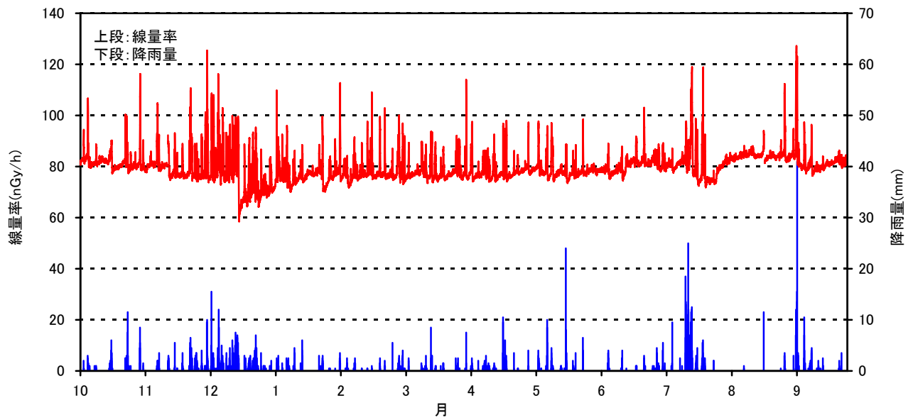
空間線量率と降雨量の測定結果(2005年 10月～2006年 9月)
