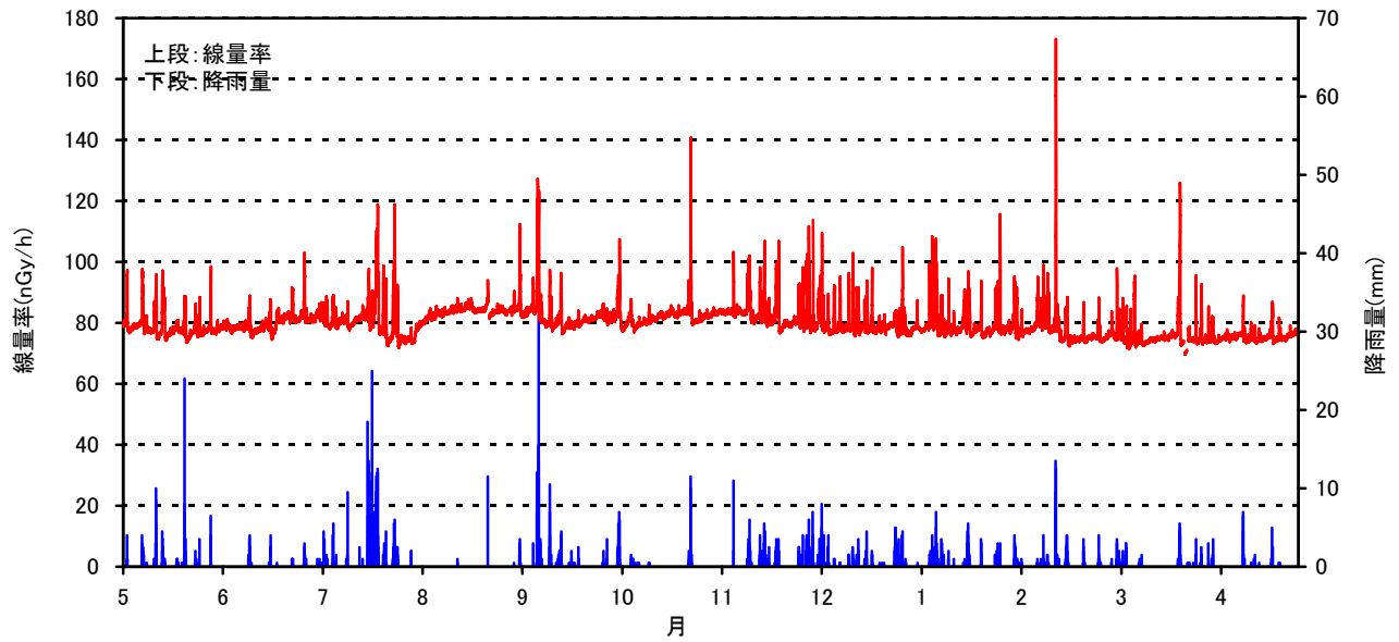
空間線量率と降雨量の測定結果(2006年 05月～2007年 4月)
