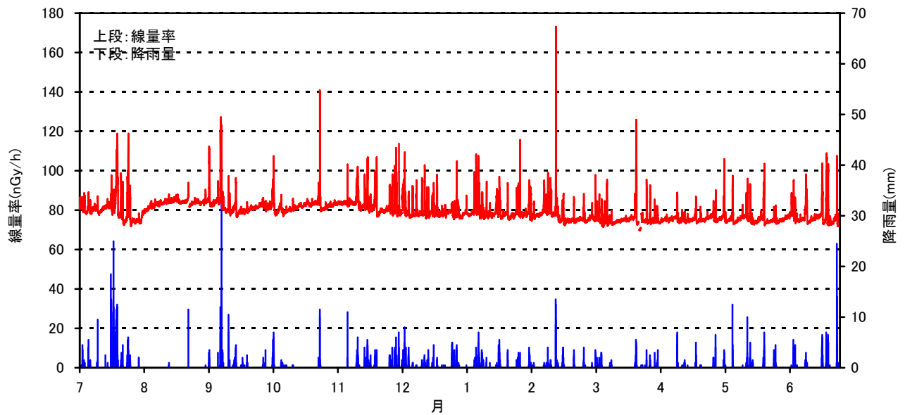
空間線量率と降雨量の測定結果(2006年 07月～2007年 6月)
