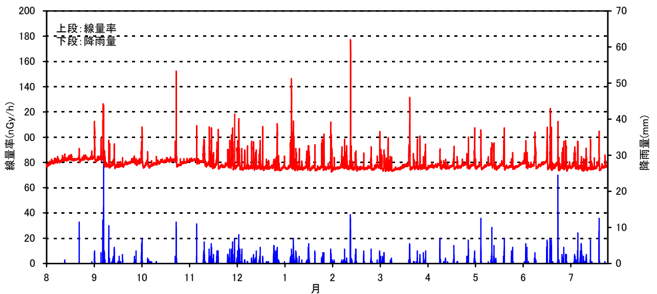
空間線量率と降雨量の測定結果(2006年 08月～2007年 7月)
