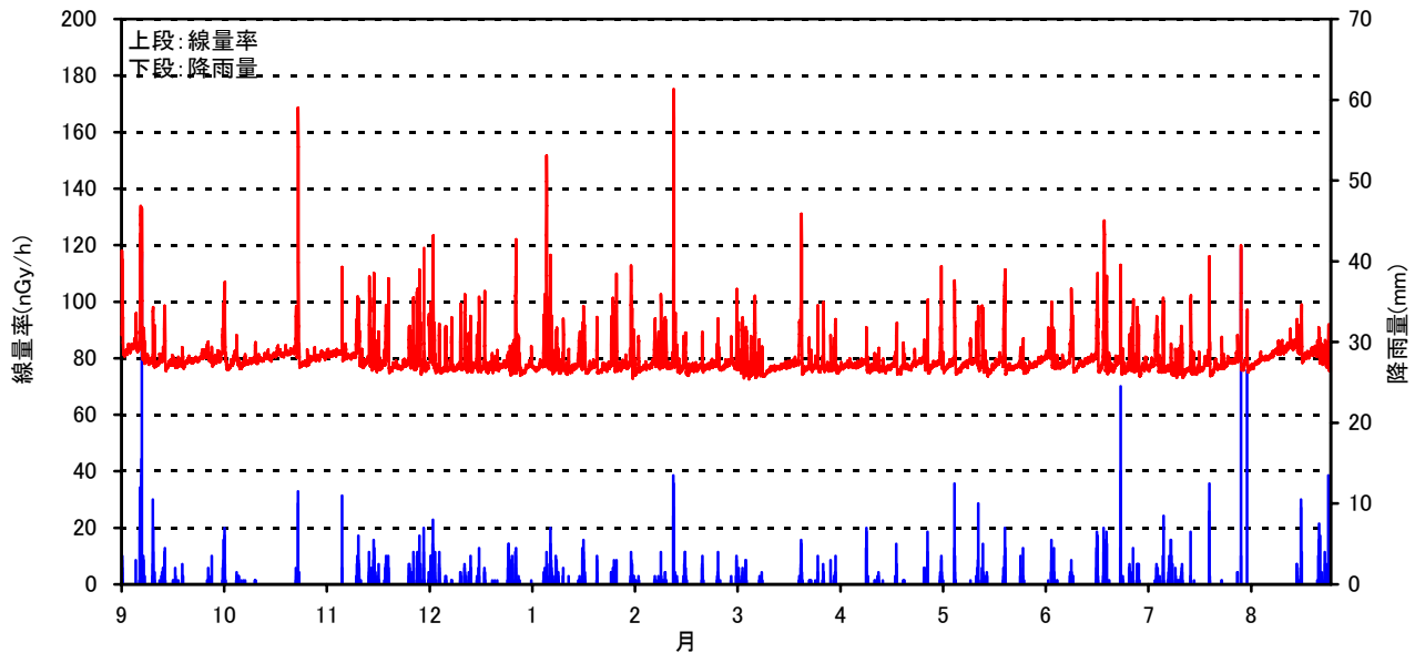
空間線量率と降雨量の測定結果(2006年 09月～2007年 8月)
