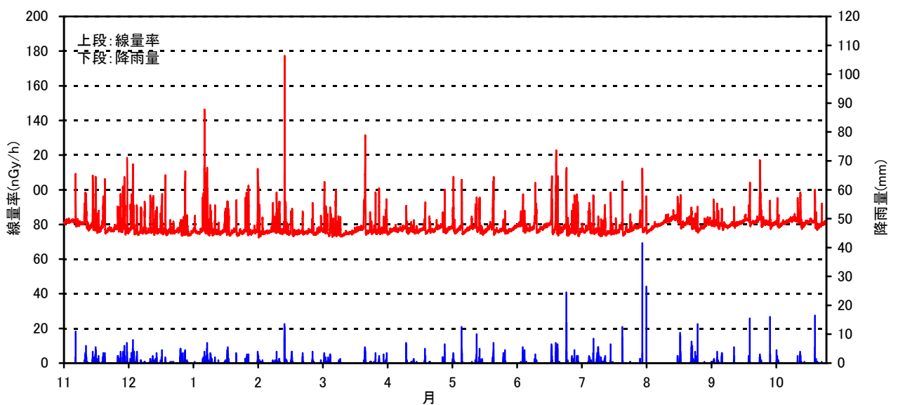
空間線量率と降雨量の測定結果(2006年 11月～2007年 10月)
