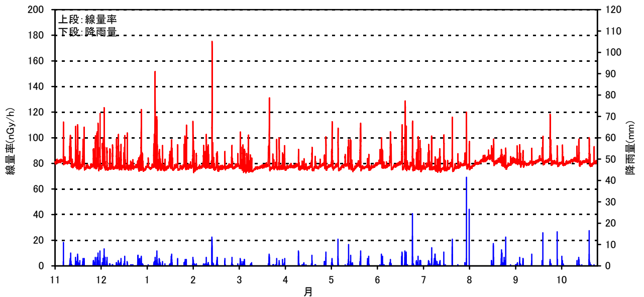
空間線量率と降雨量の測定結果(2006年 11月～2007年 10月)
