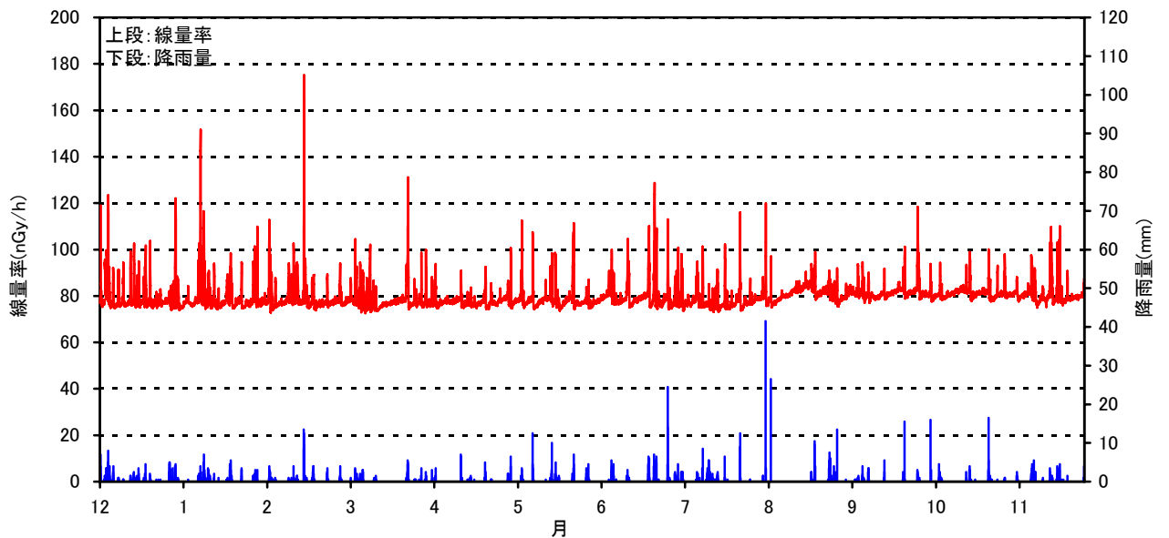
空間線量率と降雨量の測定結果(2006年 12月～2007年 11月)
