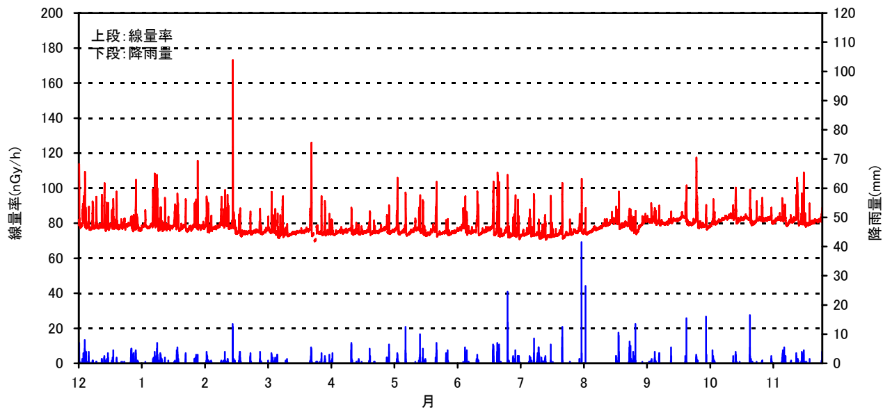
空間線量率と降雨量の測定結果(2006年 12月～2007年 11月)
