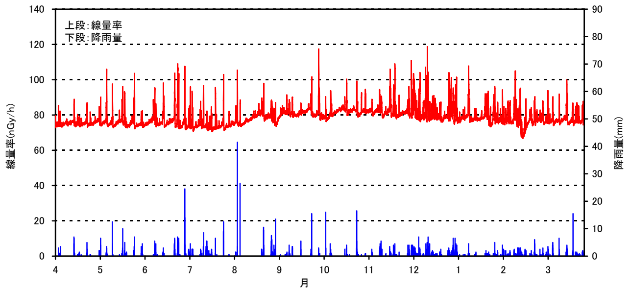
空間線量率と降雨量の測定結果(2007年 04月～2008年 3月)
