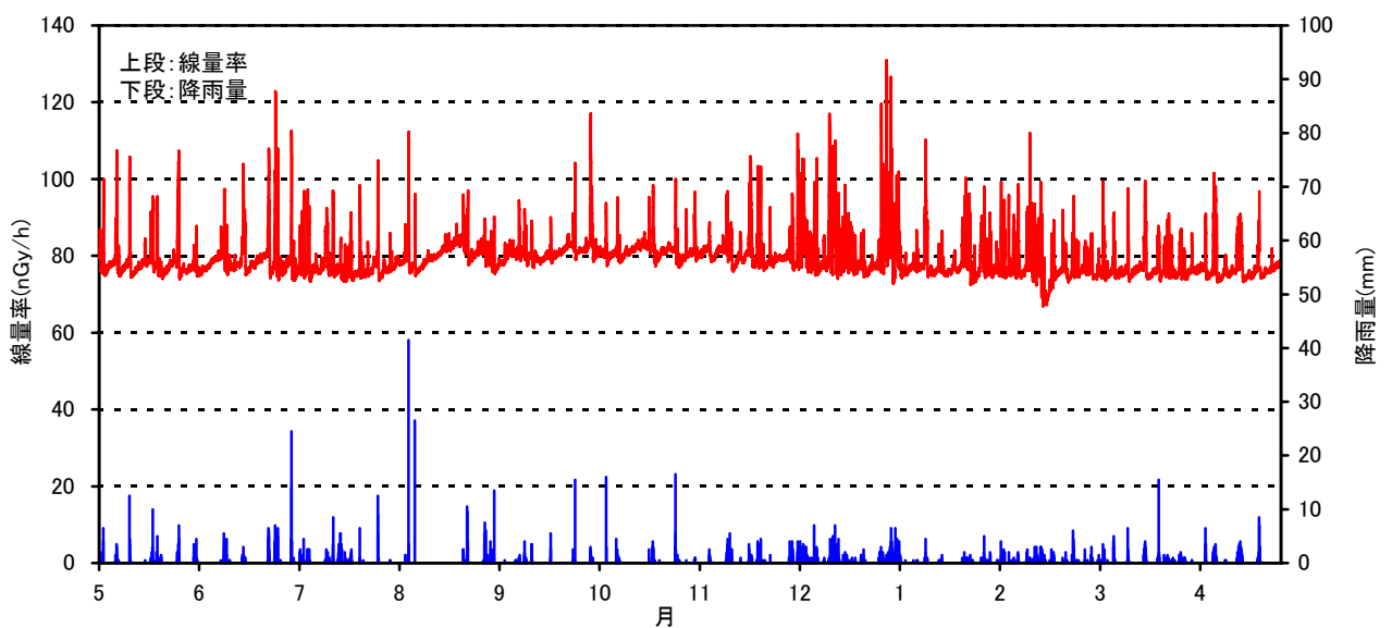
空間線量率と降雨量の測定結果(2007年 05月～2008年 4月)
