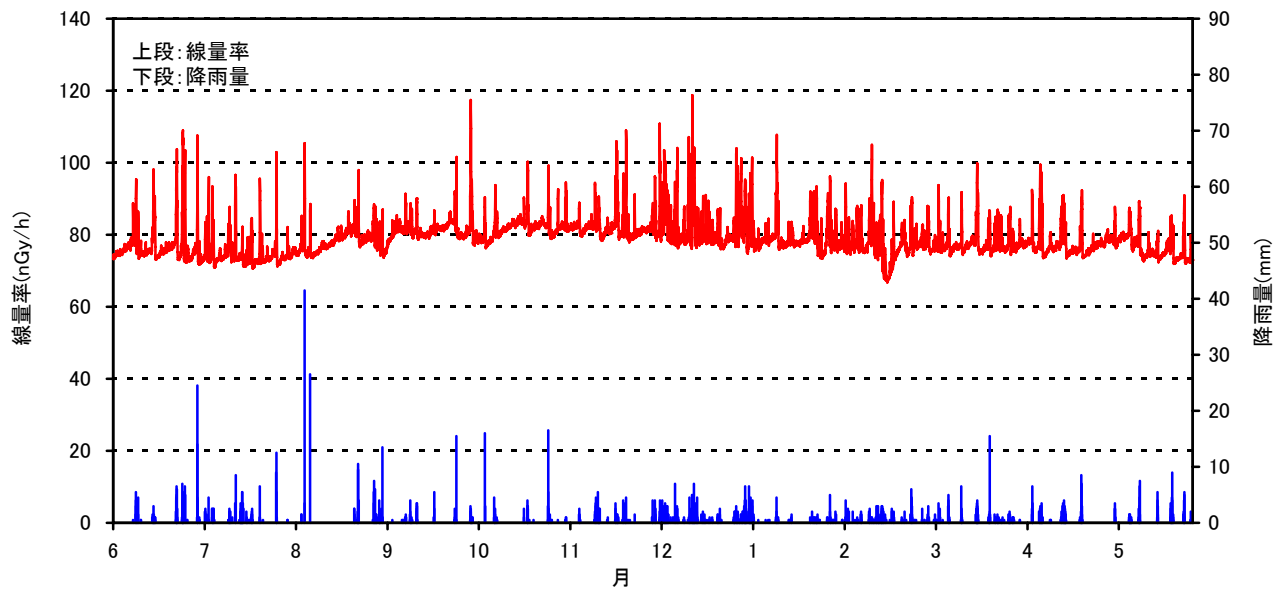
空間線量率と降雨量の測定結果(2007年 06月～2008年 5月)
