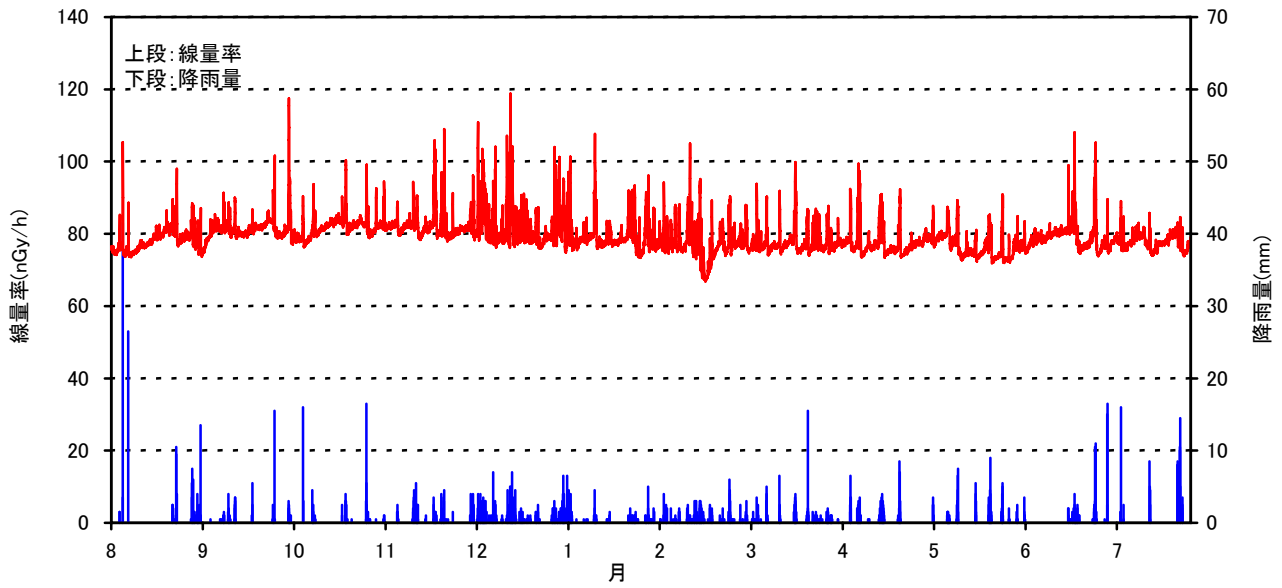
空間線量率と降雨量の測定結果(2007年 08月～2008年 7月)
