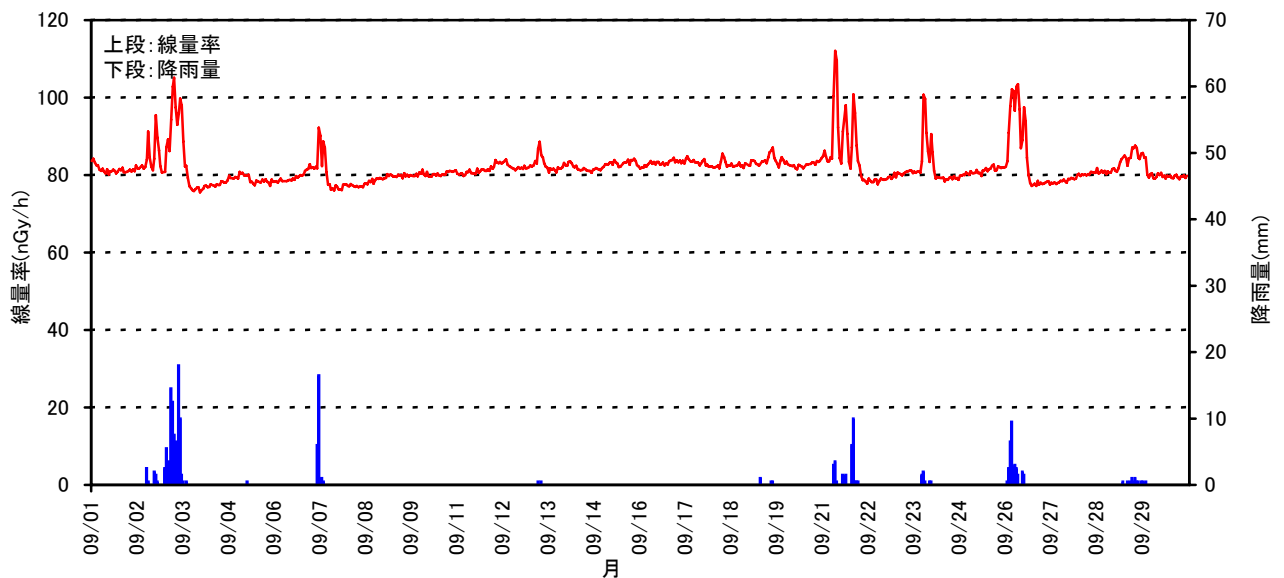
空間線量率と降雨量の測定結果(2008年 9月)
