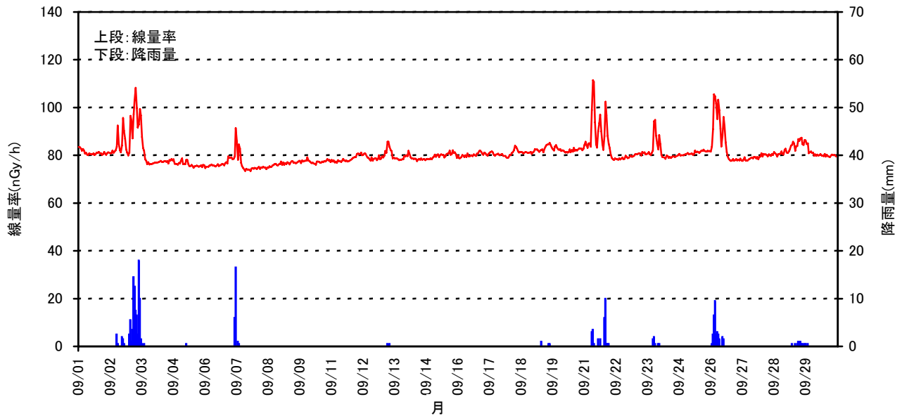
空間線量率と降雨量の測定結果(2008年 9月)
