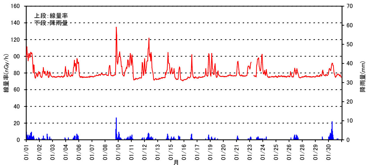
空間線量率と降雨量の測定結果(2009年 1月)
