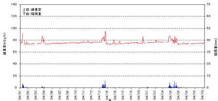
空間線量率と降雨量の測定結果(2009年 4月)
