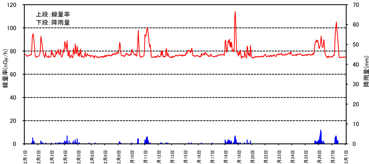
空間線量率と降雨量の測定結果(2010年 02月)
