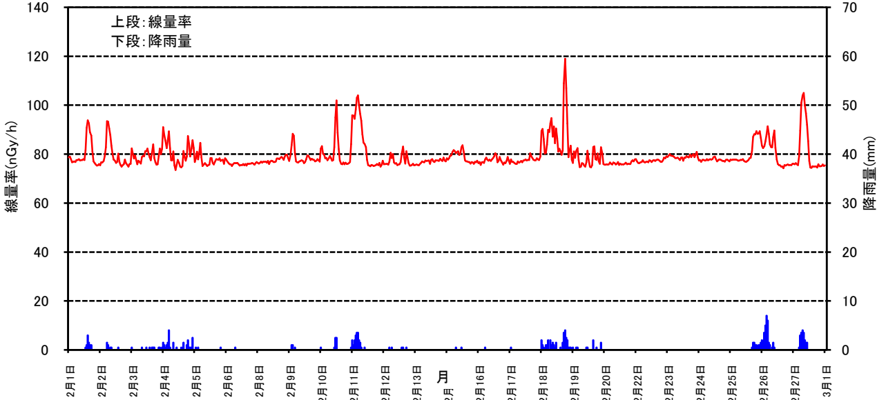
空間線量率と降雨量の測定結果(2010年 2月)
