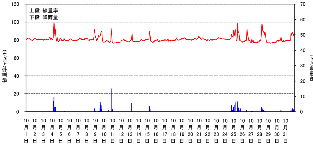
空間線量率と降雨量の測定結果(2010年 10月)
