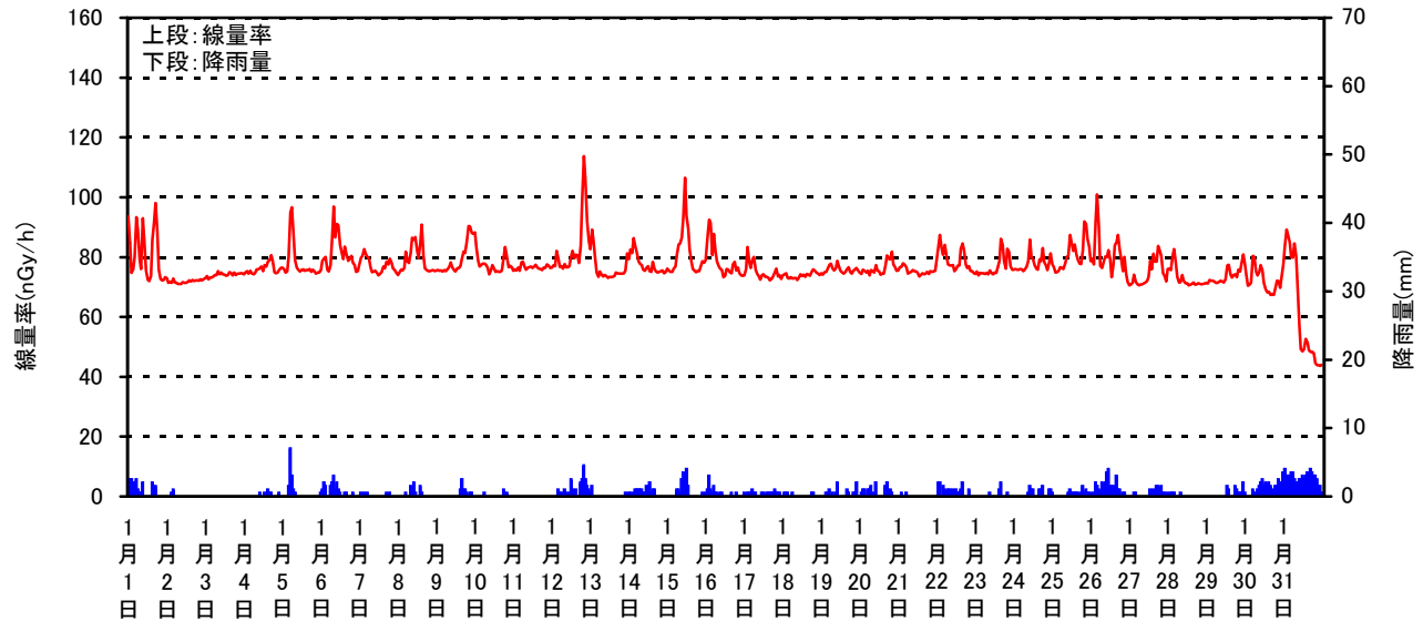
空間線量率と降雨量の測定結果(2011年 1月)
