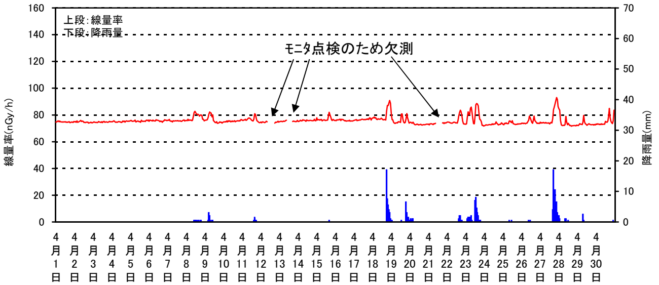
空間線量率と降雨量の測定結果(2011年 4月)
