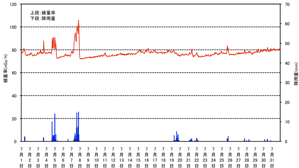
空間線量率と降雨量の測定結果(2011年 7月)
