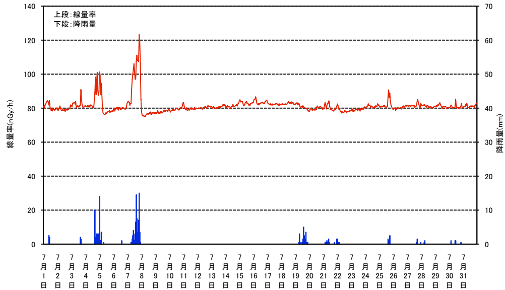
空間線量率と降雨量の測定結果(2011年 7月)
