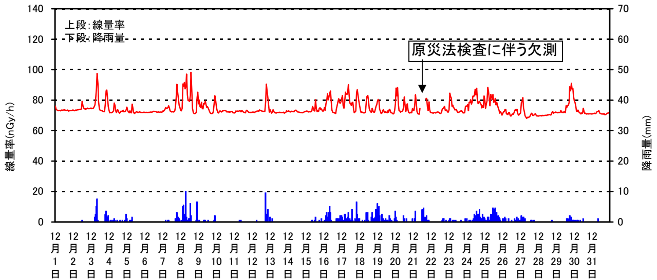
空間線量率と降雨量の測定結果(2011年 12月)
