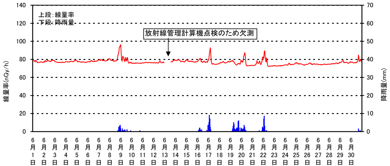
空間線量率と降雨量の測定結果(2012年 6月)
