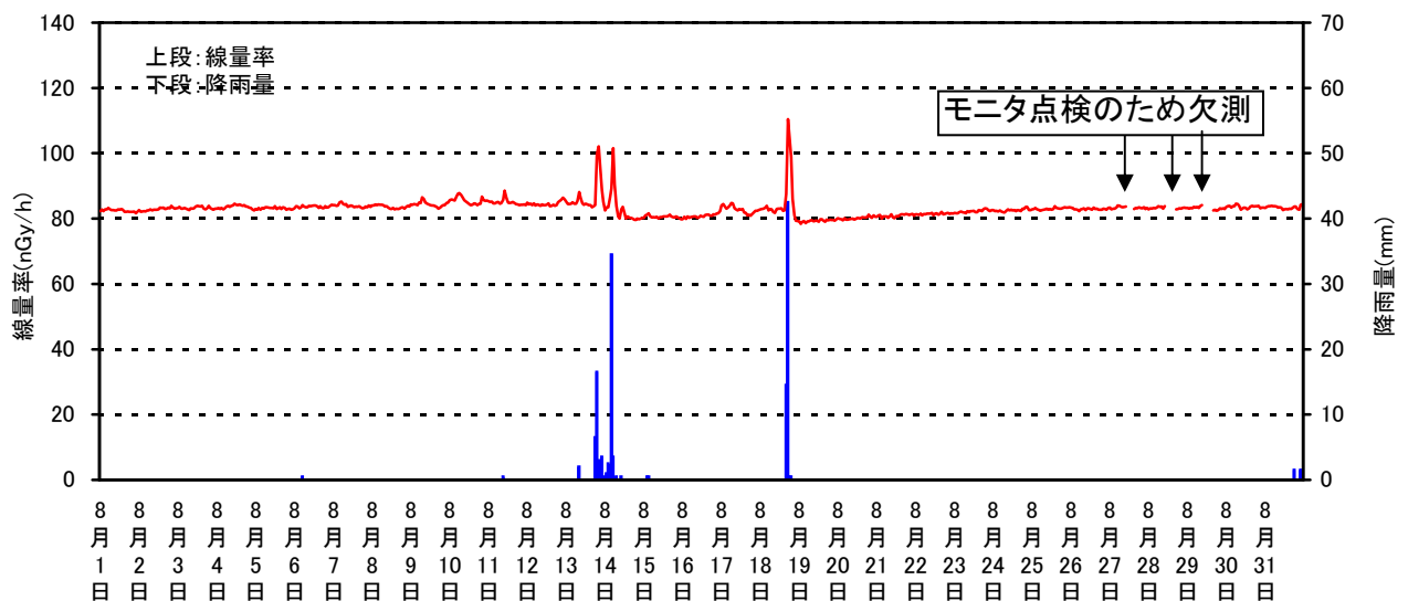
空間線量率と降雨量の測定結果(2012年 8月)
