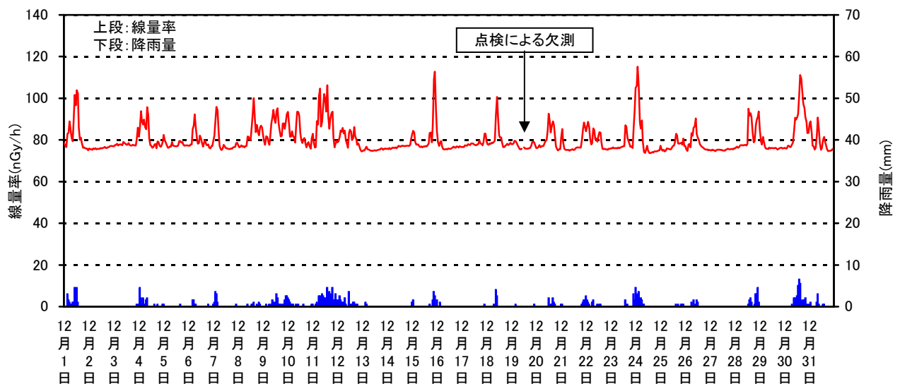
空間線量率と降雨量の測定結果(2012年12月)
