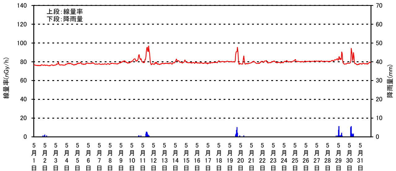
空間線量率と降雨量の測定結果(2013年5月)
