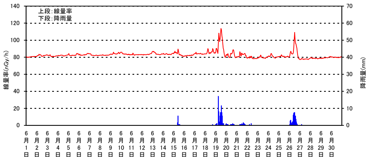
空間線量率と降雨量の測定結果(2013年6月)
