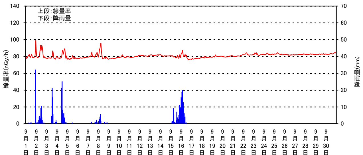
空間線量率と降雨量の測定結果(2013年9月)
