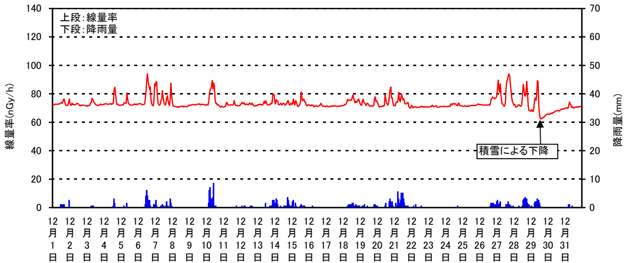
空間線量率と降雨量の測定結果(2013年12月)
