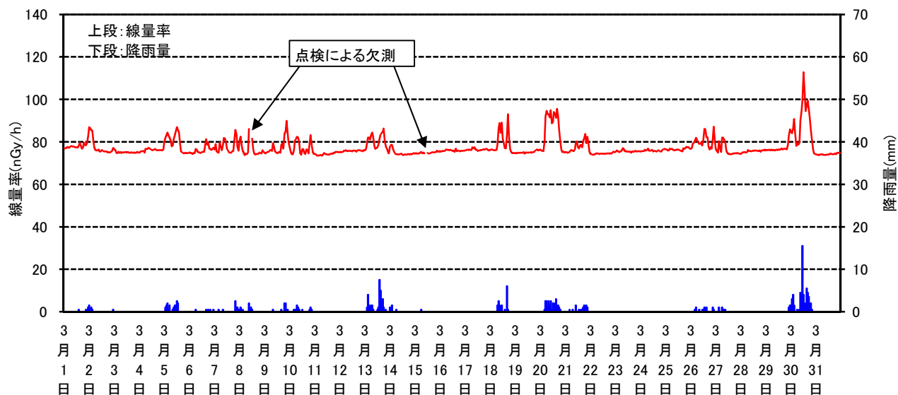
空間線量率と降雨量の測定結果(2014年3月)
