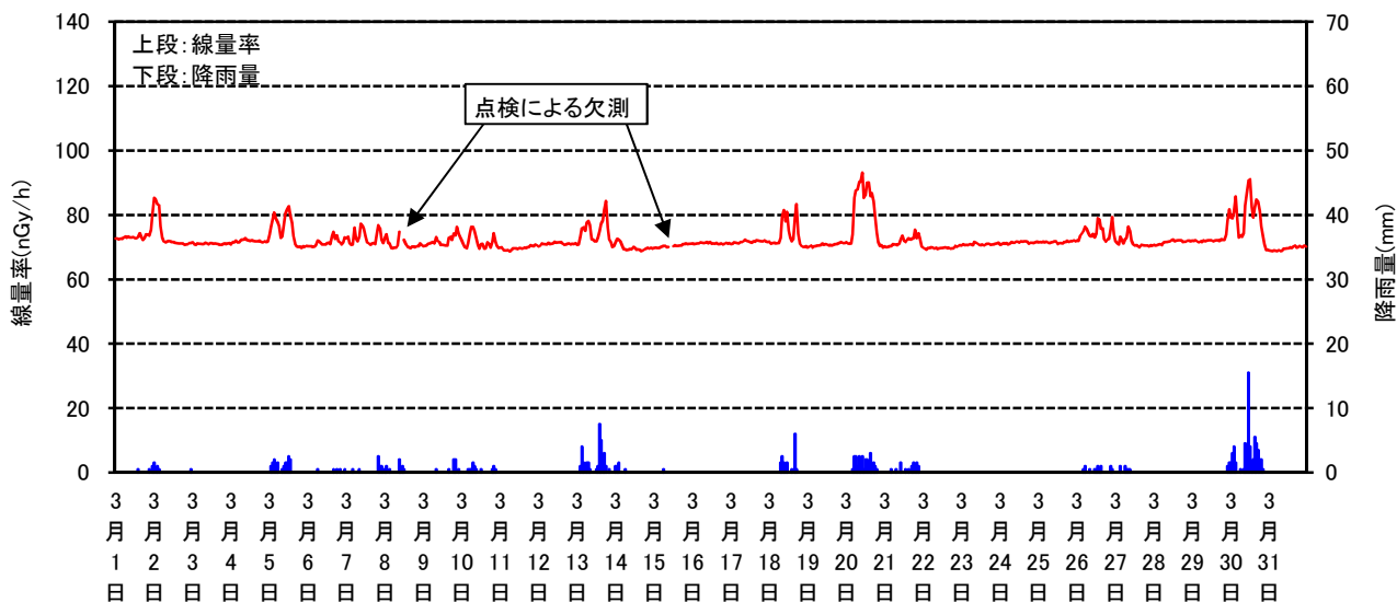
空間線量率と降雨量の測定結果(2014年3月)
