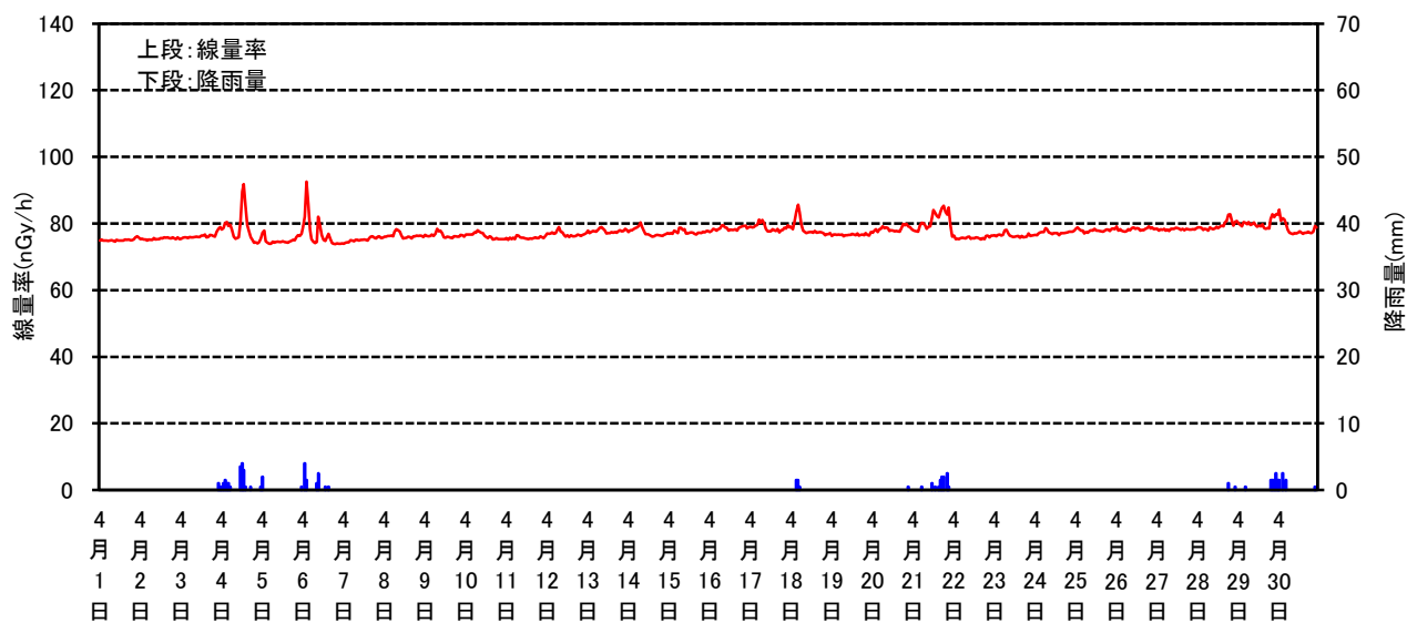
空間線量率と降雨量の測定結果(平成26年4月)
