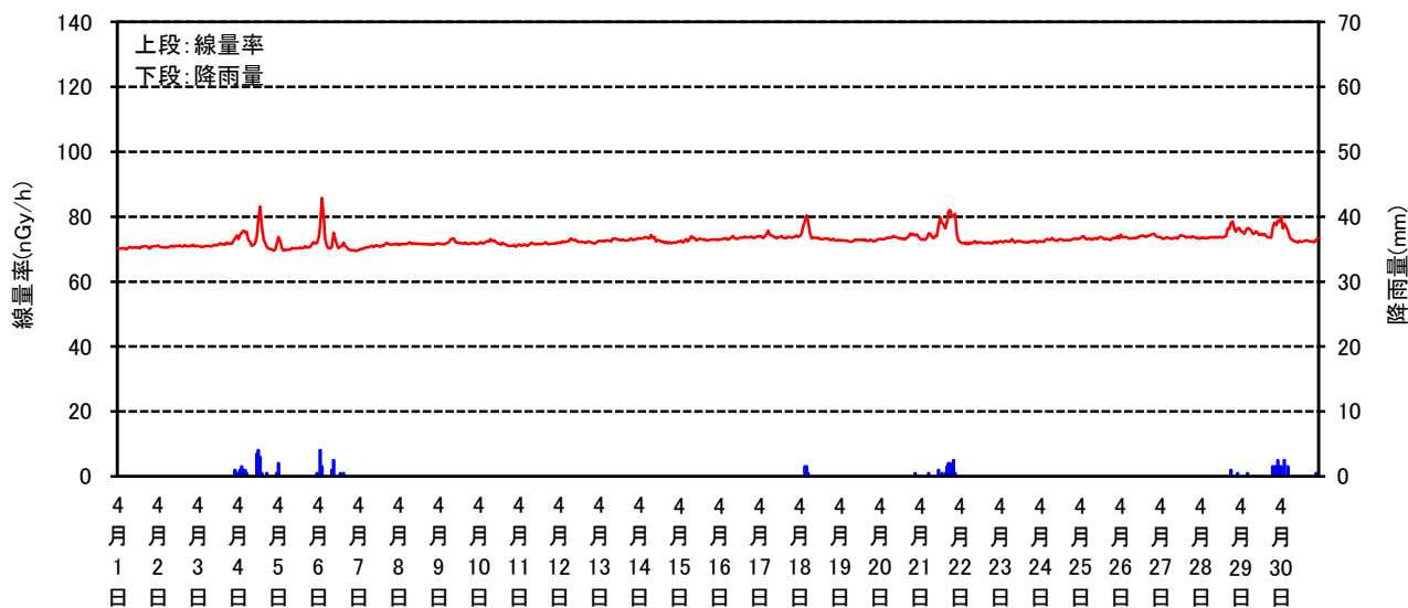
空間線量率と降雨量の測定結果(平成26年4月)
