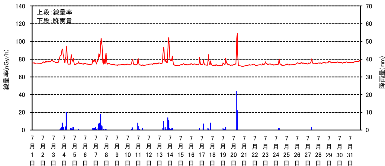
空間線量率と降雨量の測定結果(平成26年7月)
