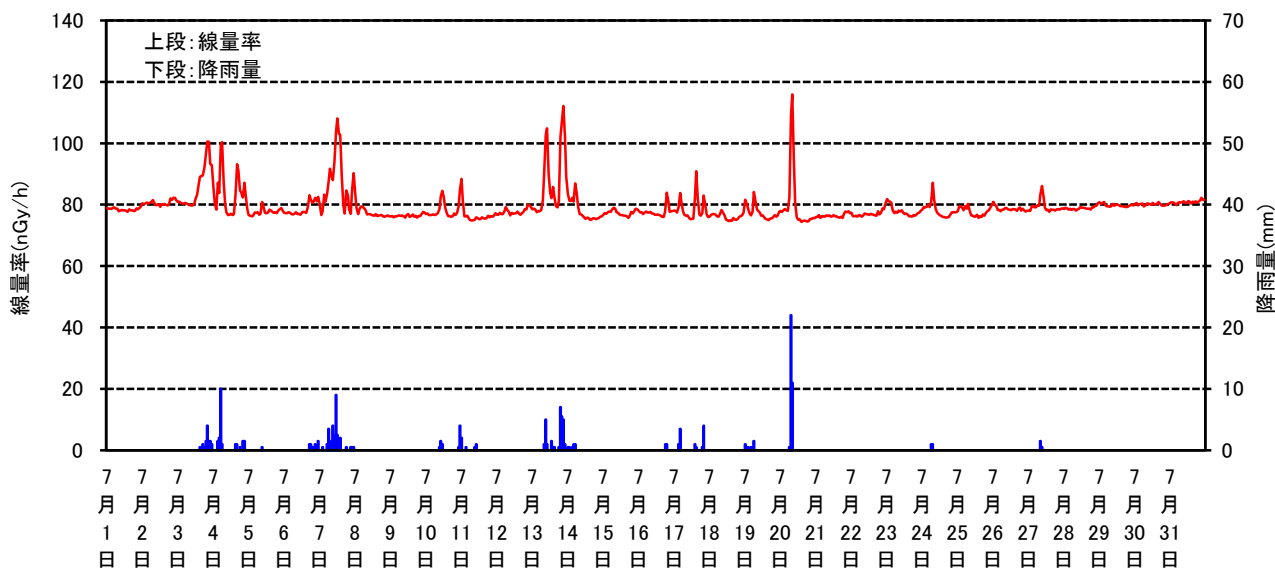
空間線量率と降雨量の測定結果(平成26年7月)
