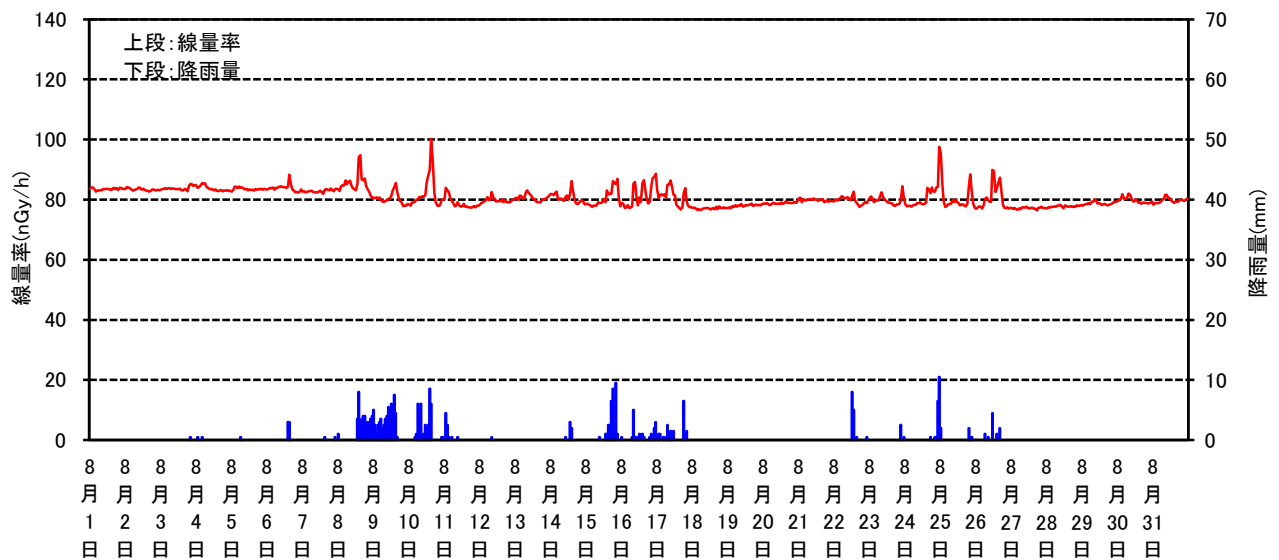
空間線量率と降雨量の測定結果(平成26年8月)
