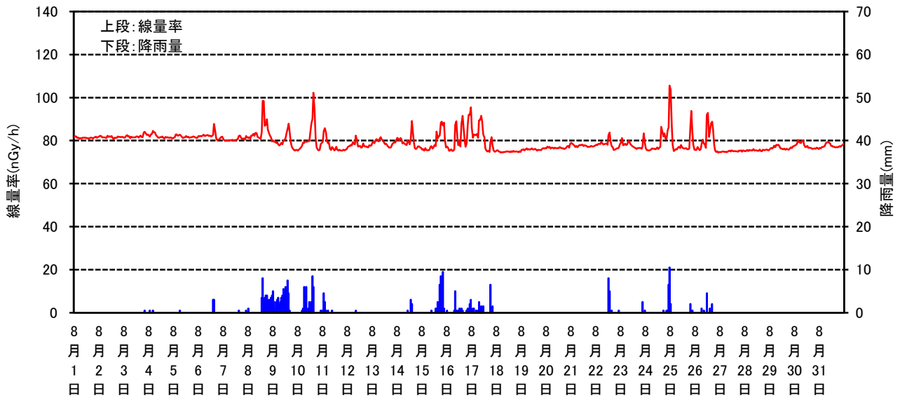
空間線量率と降雨量の測定結果(平成26年8月)
