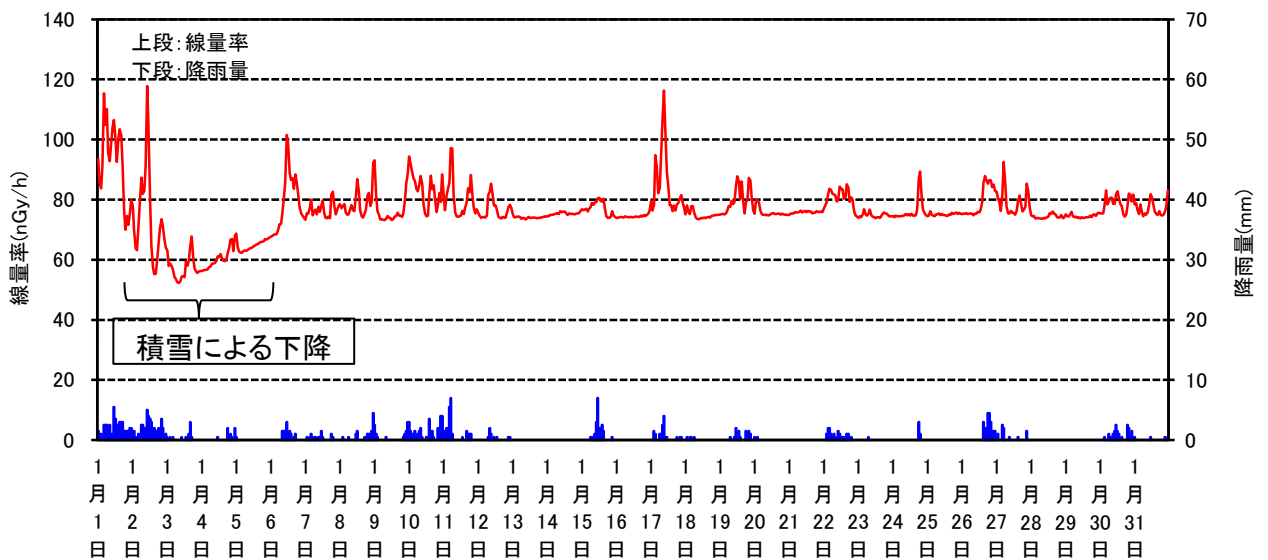
空間線量率と降雨量の測定結果(平成27年1月)
