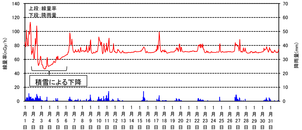
空間線量率と降雨量の測定結果(平成27年1月)
