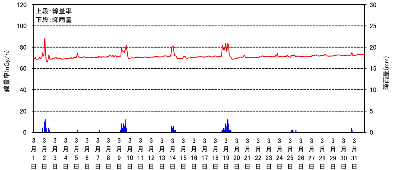
空間線量率と降雨量の測定結果(平成28年3月)
