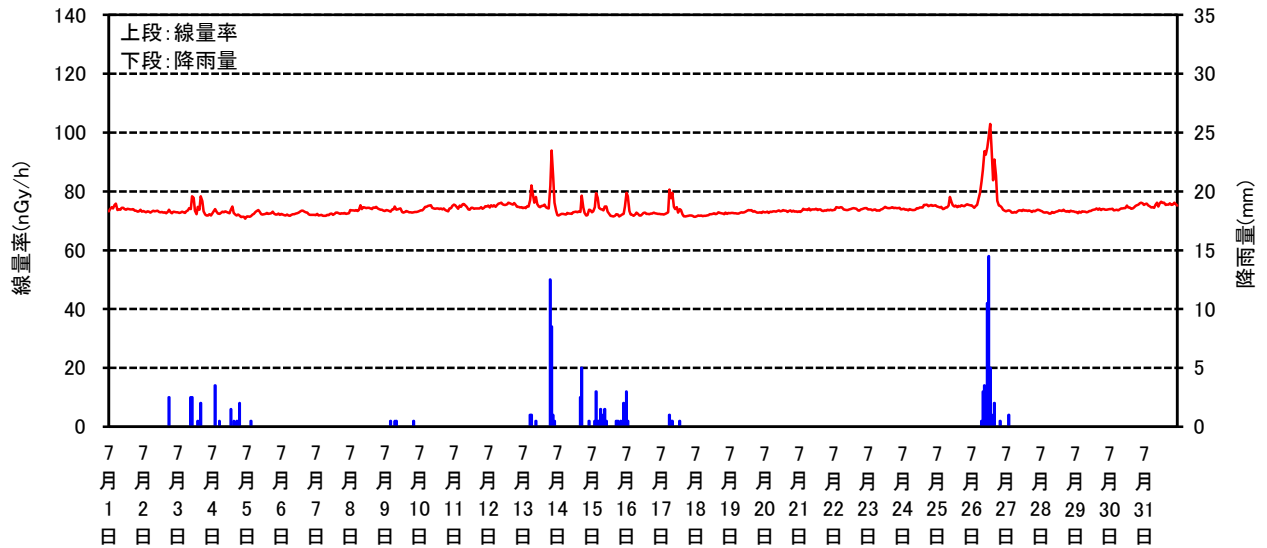
空間線量率と降雨量の測定結果(平成28年7月)
