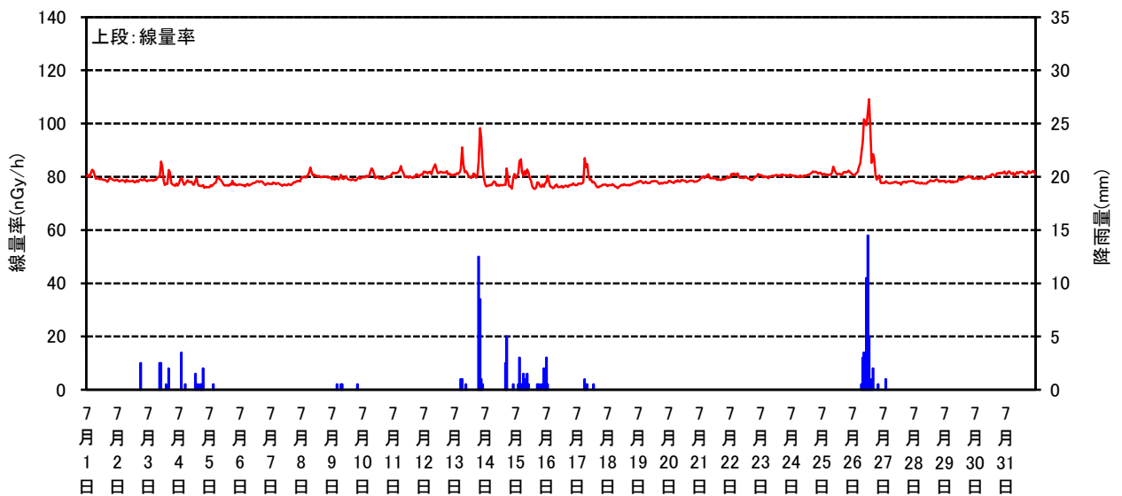
空間線量率と降雨量の測定結果(平成28年7月)
