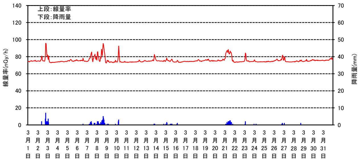
空間線量率と降雨量の測定結果(平成29年03月)
